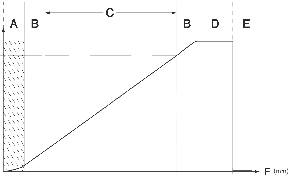
Ausgangskennlinie Analogausgang
