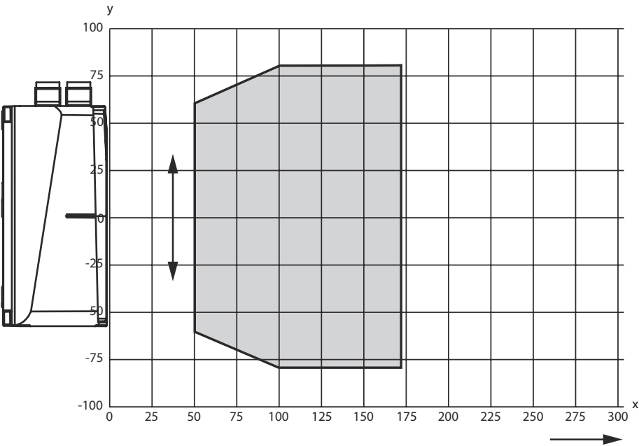
Lesefeldkurve
