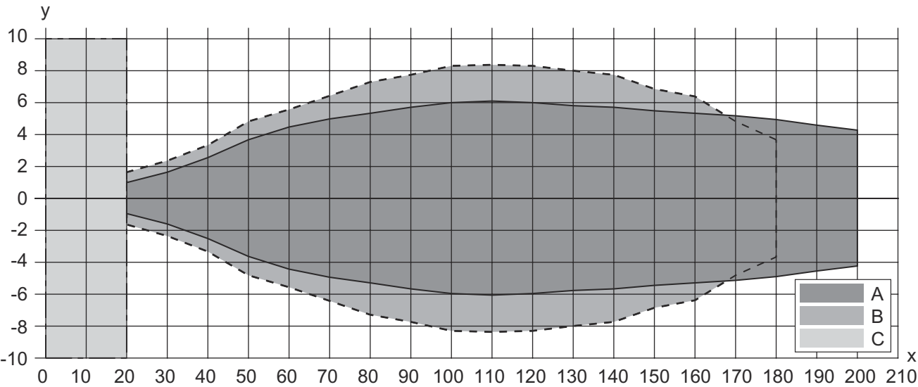
Typisch aanspreekgedrag
