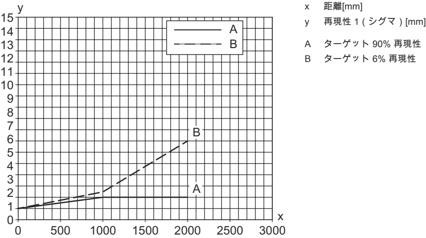
S/W エラーダイアグラム
