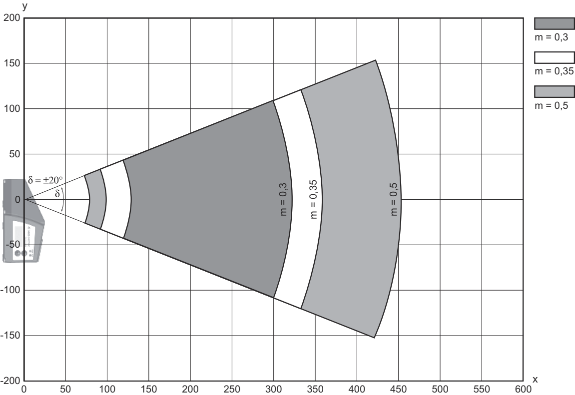
侧面条码阅读曲线
