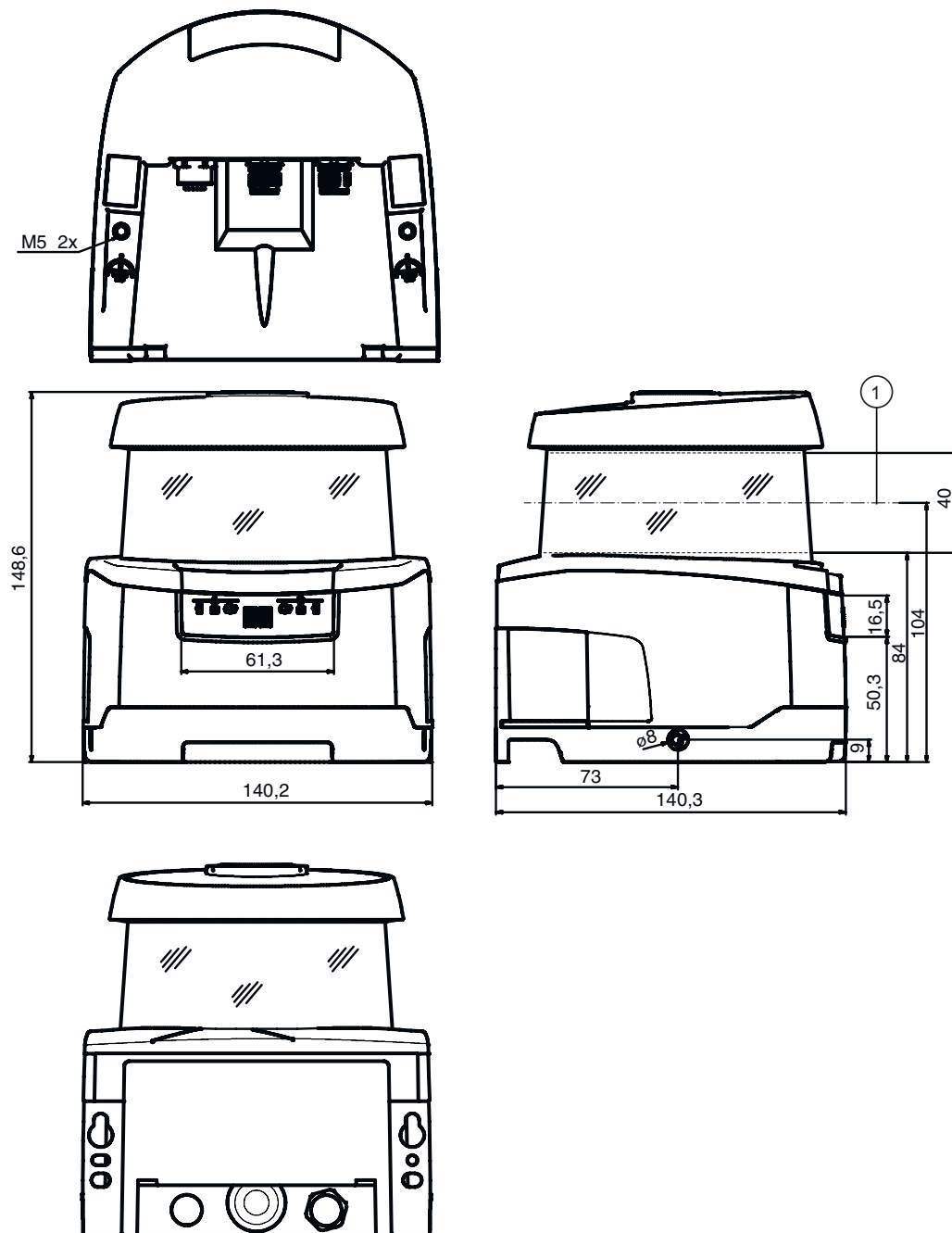
1 Płaszczyzna skanowania
