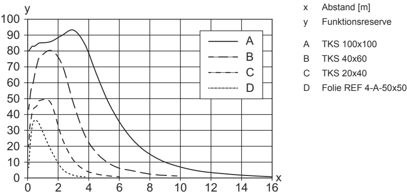
Typ. Funktionsreserve
