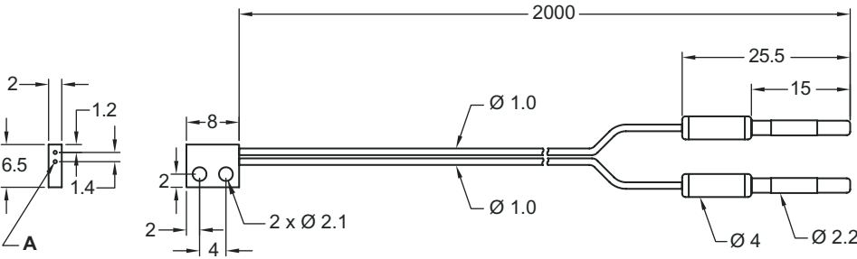
A Ø 0.5 mm 塑料纤维芯 x 2 件
