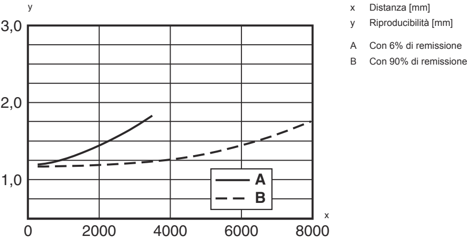
Riproducibilità tip. modalità di misura «Standard»
