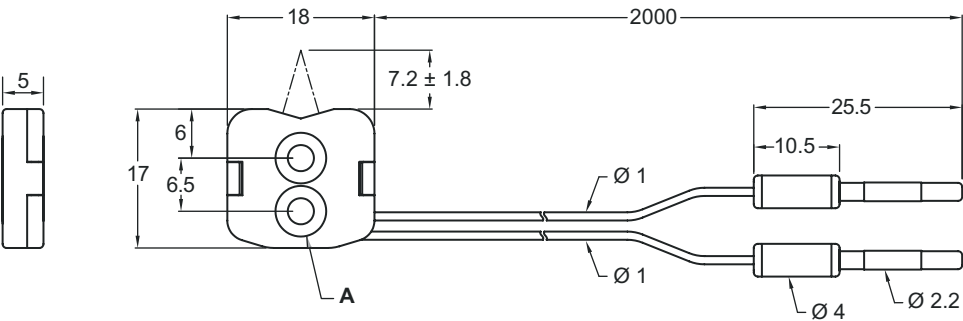
A 2 x Ø 3,2 / Ø 6,2 (foro di montaggio, lato frontale)
