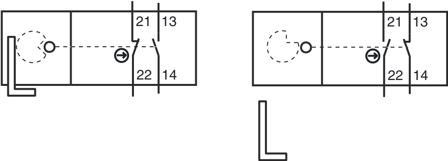
21/22 Styk normalnie zamknięty (NC) z wymuszonym prowadzeniem
