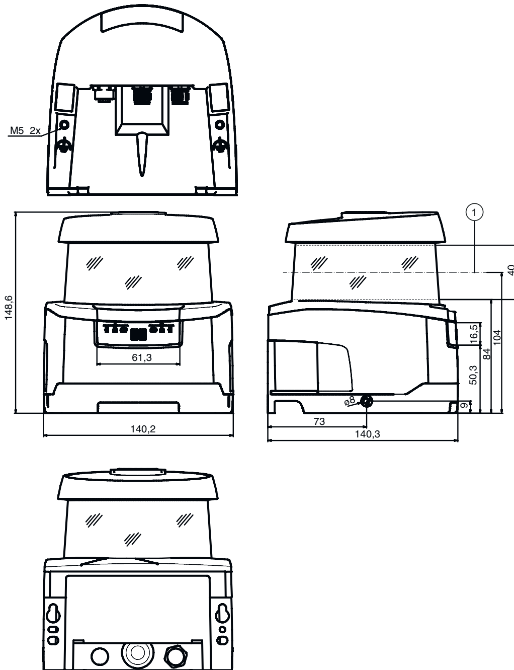
1 扫描平面
