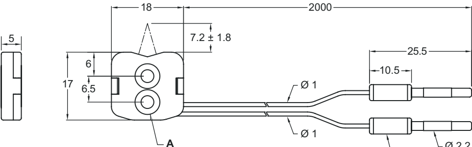
A 2 x Ø 3.2 / Ø 6.2 ( 正面装配孔 )
