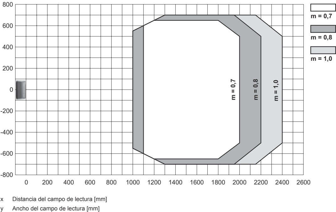
Curva del campo de lectura
