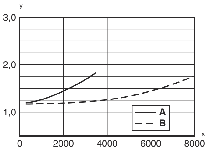
Typ. reproduceerbaarheid meetmodus "Nauwkeurigheid"
