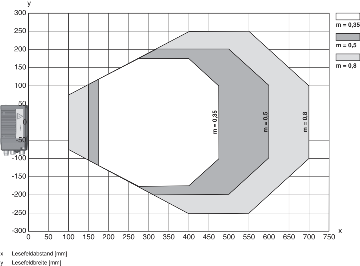
Lesefeldkurve
