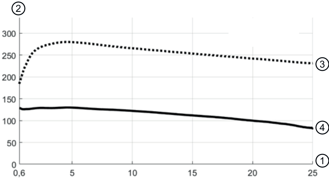
Curvas de la potencia de señal en función de la distancia
