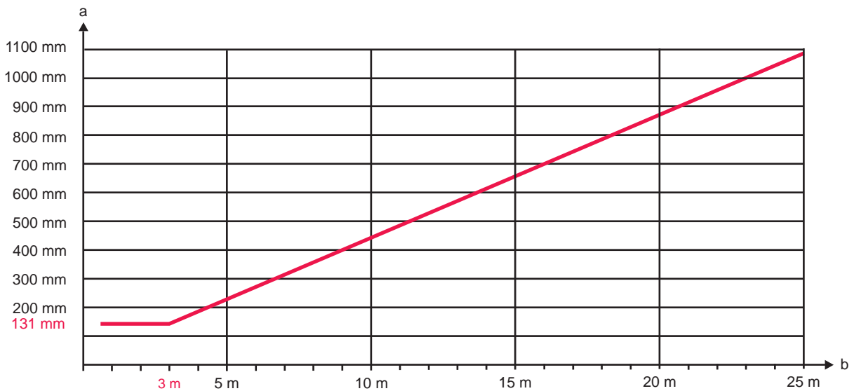
Figura 5.2: Distancia mínima respecto a las superficies reflectantes según la anchura del campo de protección
