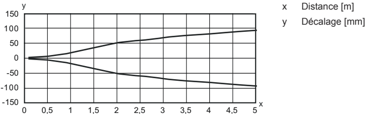
Réaction typ. (TKS100x100)
