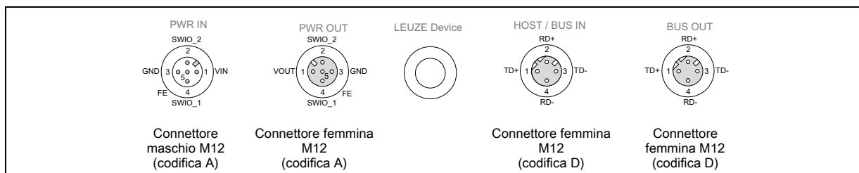
Figura 12.1: Collegamenti dell'MA 208 i visti da sotto, dispositivo su piastra di montaggio
