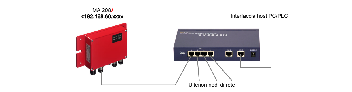
Figura 4.4: Ethernet nella topologia a stella
