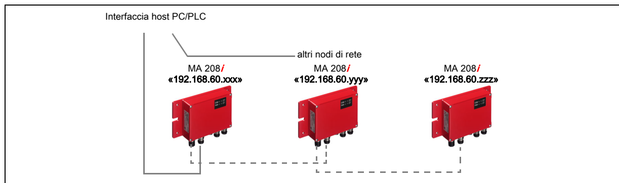
Figura 4.5: Ethernet nella topologia lineare
