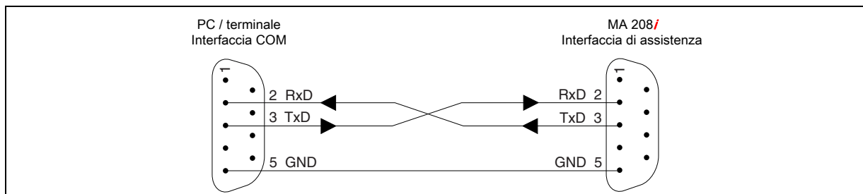
Figura 7.7: Collegamento dell'interfaccia di assistenza ad un PC/terminale
