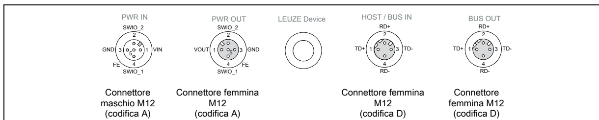
Figura 3.1: Collegamenti dell'MA 208 i
