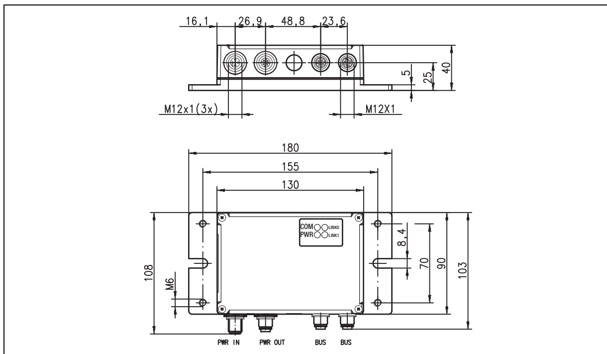
Figura 5.1: Disegno quotato MA 208 i
