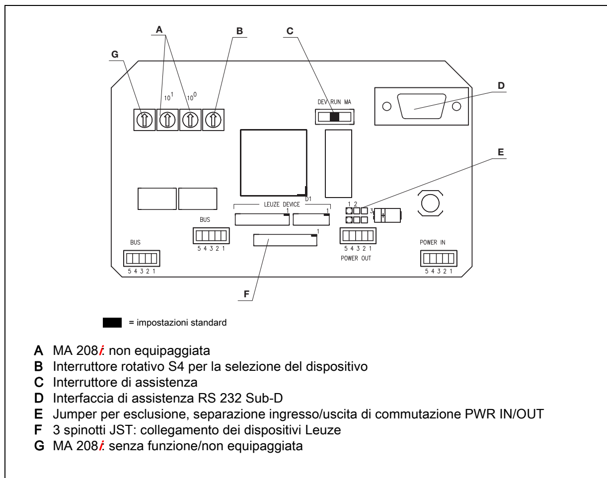
Figura 8.2: Vista anteriore: elementi di controllo dell'MA 208 i
