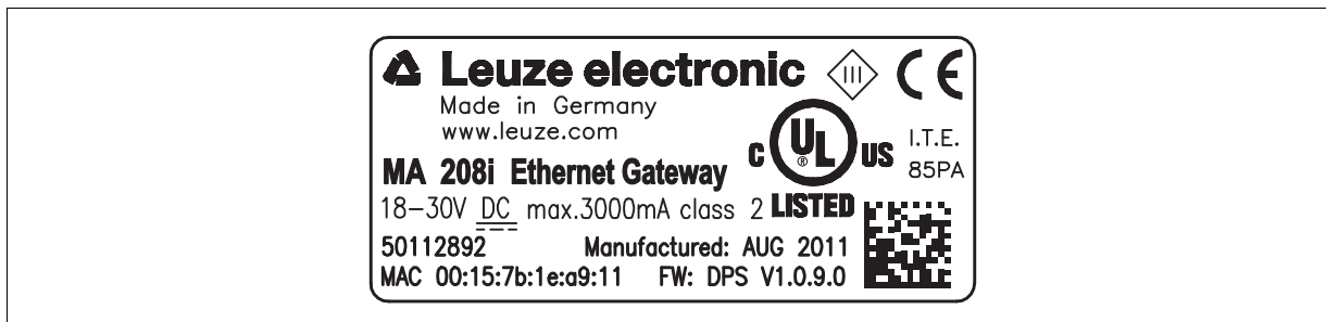
Figura 6.1: Targhetta del dispositivo MA 208/i
