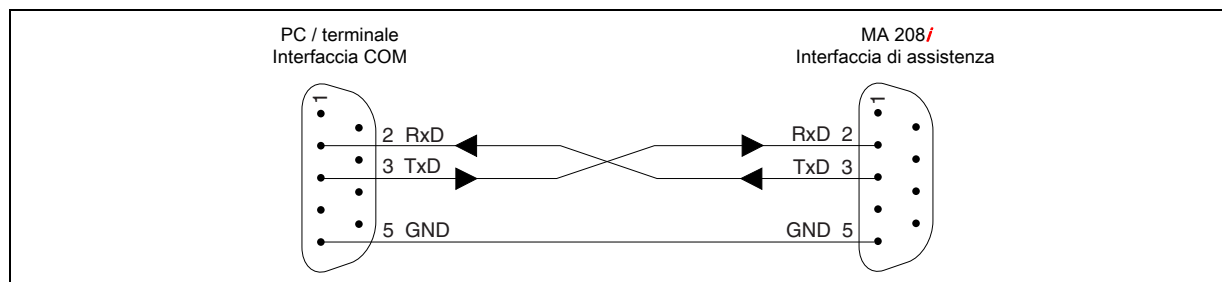
Figura 4.3: Collegamento dell'interfaccia di assistenza ad un PC/terminale
