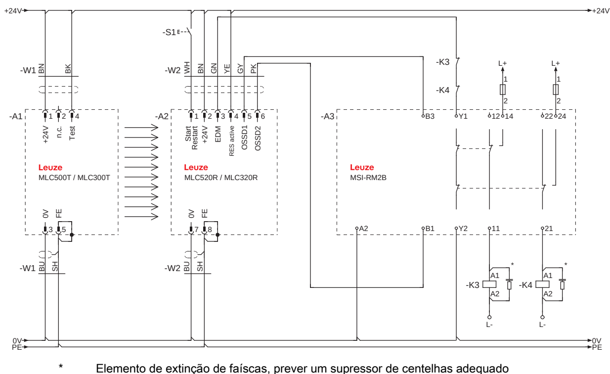
Ilustração 7.1: Relé de segurança MSI-RM2B com cortina de luz de segurança MLC 500 / MLC 300
