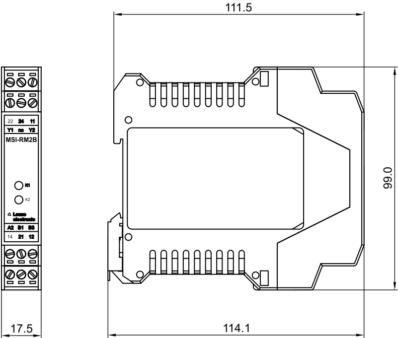
Ilustração 13.1: Dimensões MSI-RM2B-01
