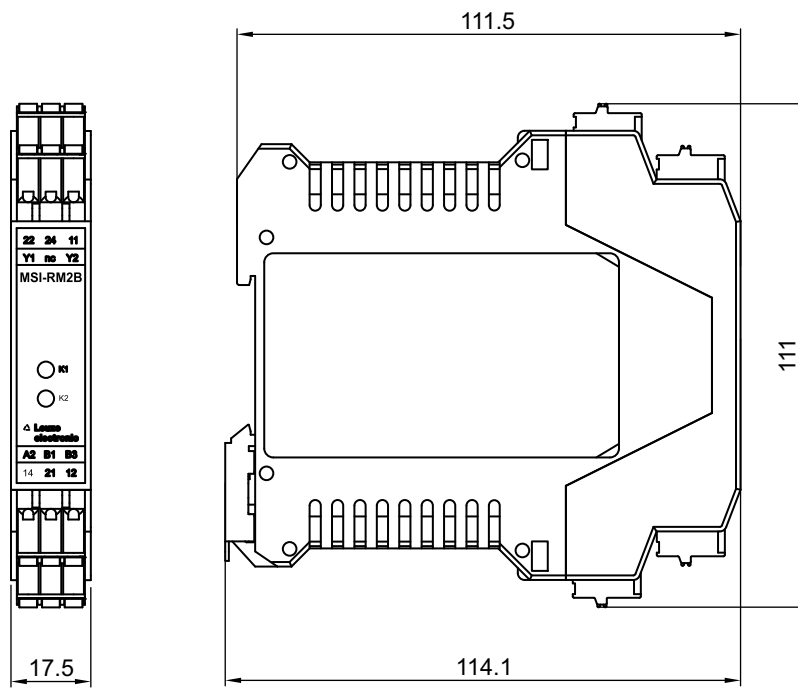
Ilustração 13.2: Dimensões MSI-RM2B-02
