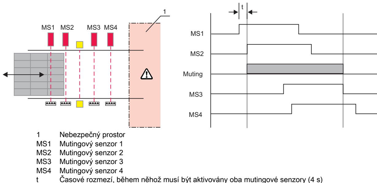
Obrázek 4.5: Časové řízený 4senzorový muting: uspořádání mutingových senzorů a časový průběh
