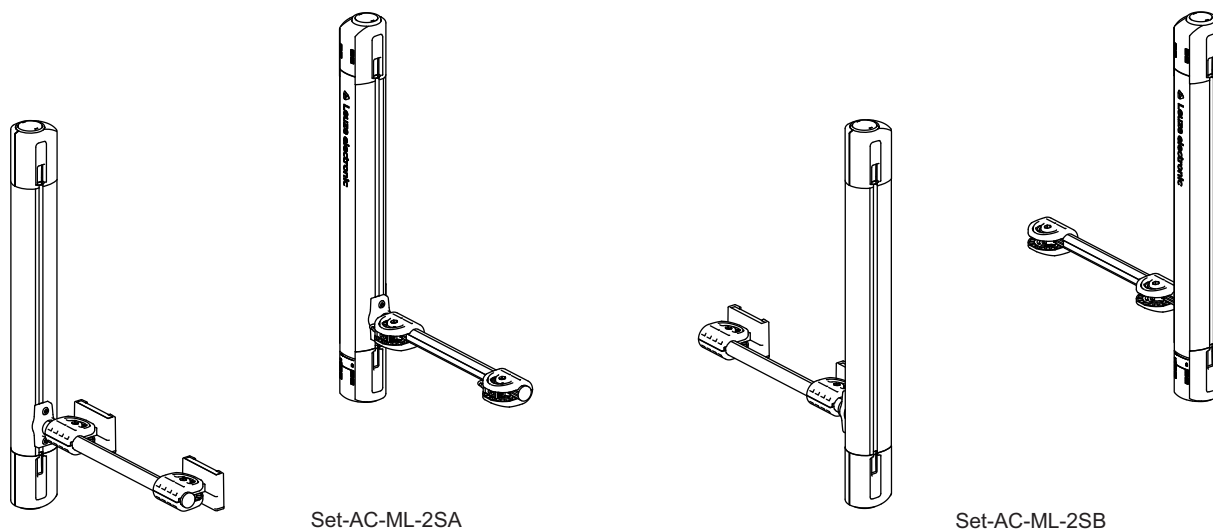
Obrázek 14.15: Sada AC-ML-2SA resp. Sada AC-ML-2SB montované na víceprskové bezpečnostní světelné závory MLD 500
