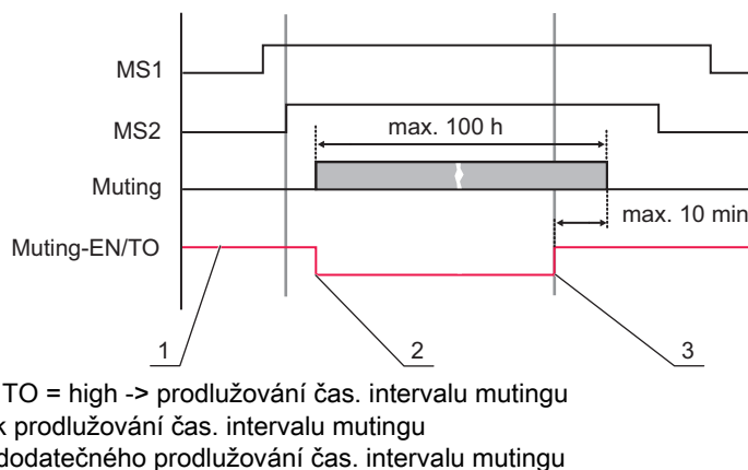
Obrázek 4.6: Prodloužení čas. intervalu mutingu
