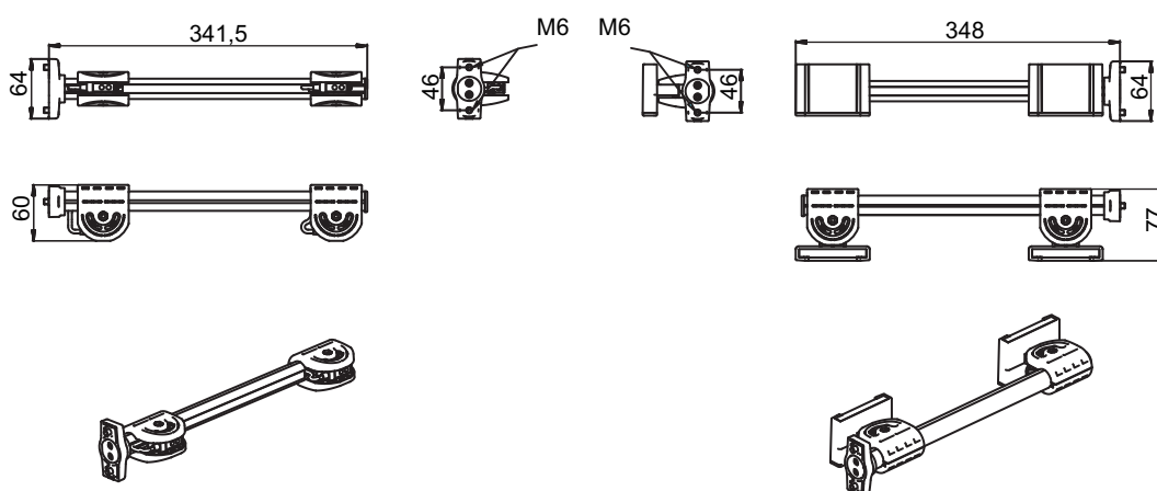
Obrázek 14.16: Sada mutingových senzorů, časově řízený 4senzorový muting
