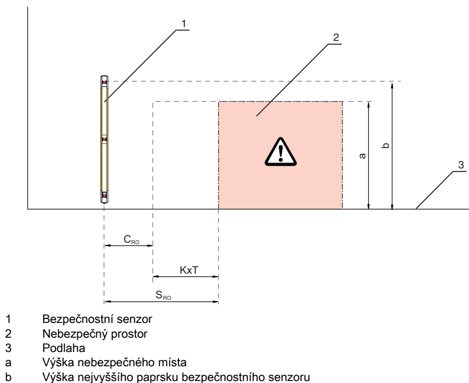
Obrázek 6.2: Navýšení bezpečnostního odstup u přesáhnutí a protažení se pod polem
