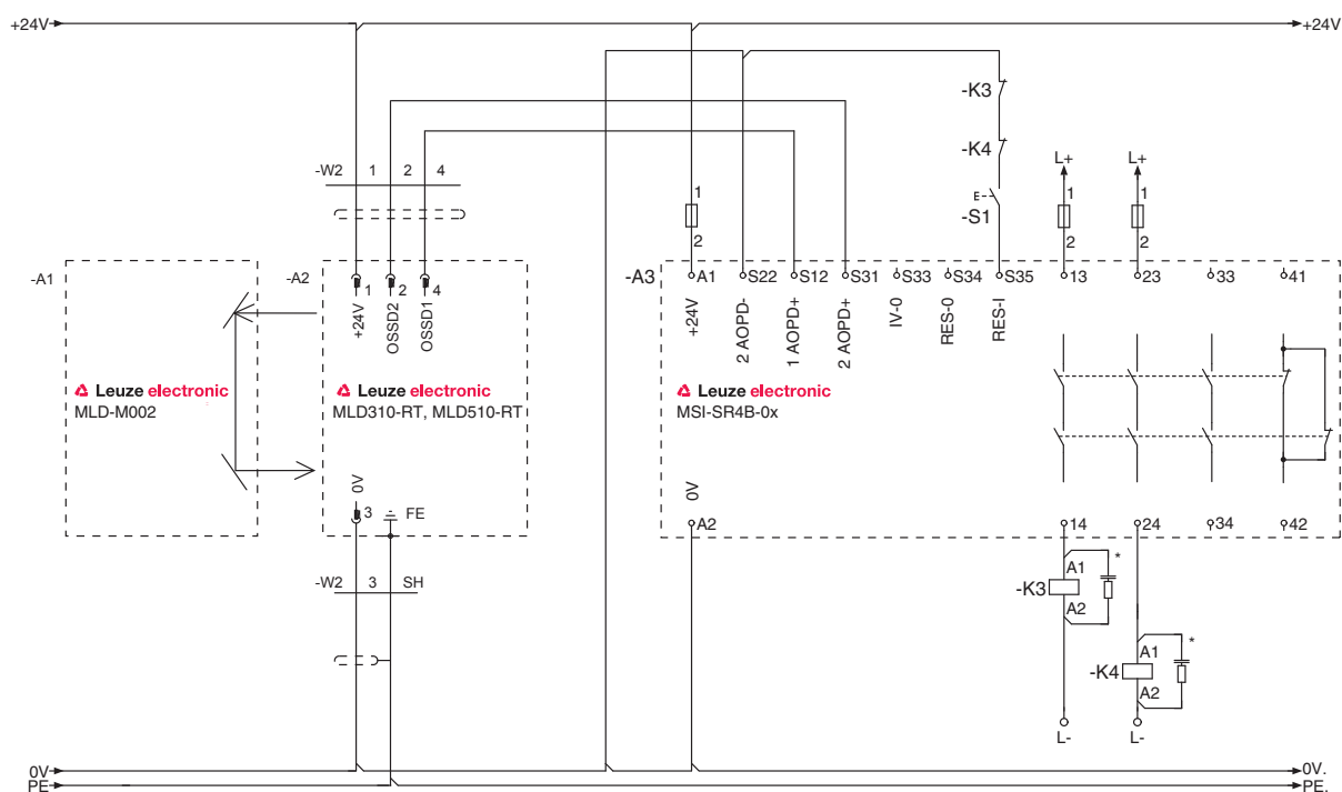
Obrázek 7.8: Příklad připojení MLD 510 (transceiverový systém) s EDM; RES v bezpečnostním spínacím přístroji MSI-SR4B-0x
