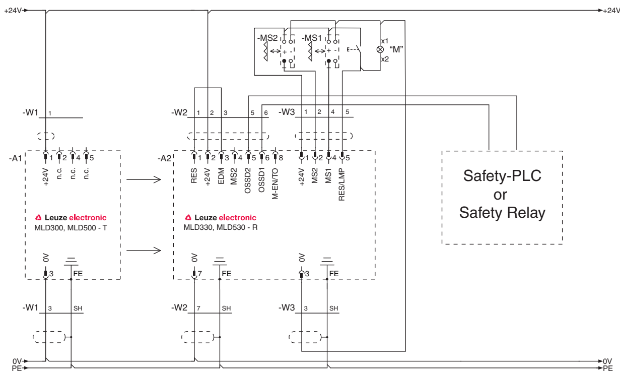
Obrázek 7.16: Příklad připojení MLD 330, MLD 530 (systém typu vysílač-přijímač): Sekvenčně řízený 2senzorový muting s čas. intervalem mutingu 100 h (připojení transceiveru obdobně k tomuto)
