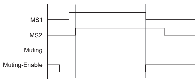
Obrázek 4.10: Bez platného signálu povolení (Enable) mutingu
