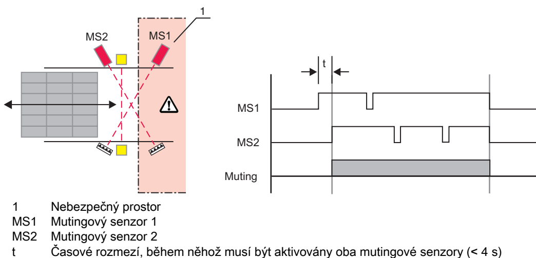
Obrázek 4.2: Časově řízený 2senzorový muting – uspořádání mutingových senzorů a časový průběh
