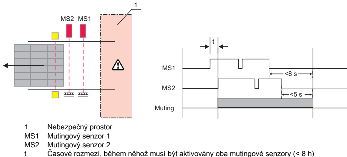
Obrázek 4.3: Sekvenčně řízený 2senzorový muting – uspořádání mutingových senzorů a časový průběh
