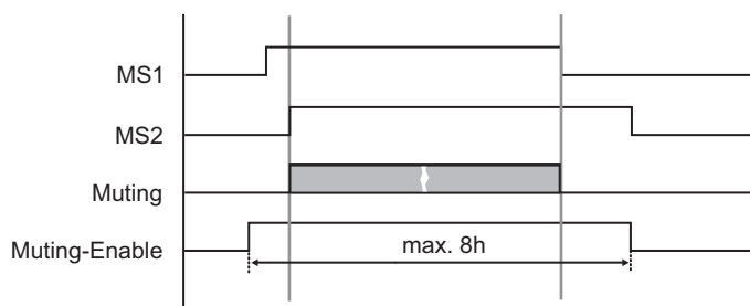
Obrázek 4.9: Povolení (Enable) mutingu
