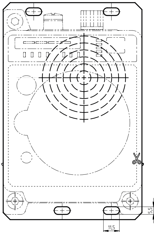
Bild 4.1: Bohrschablone
