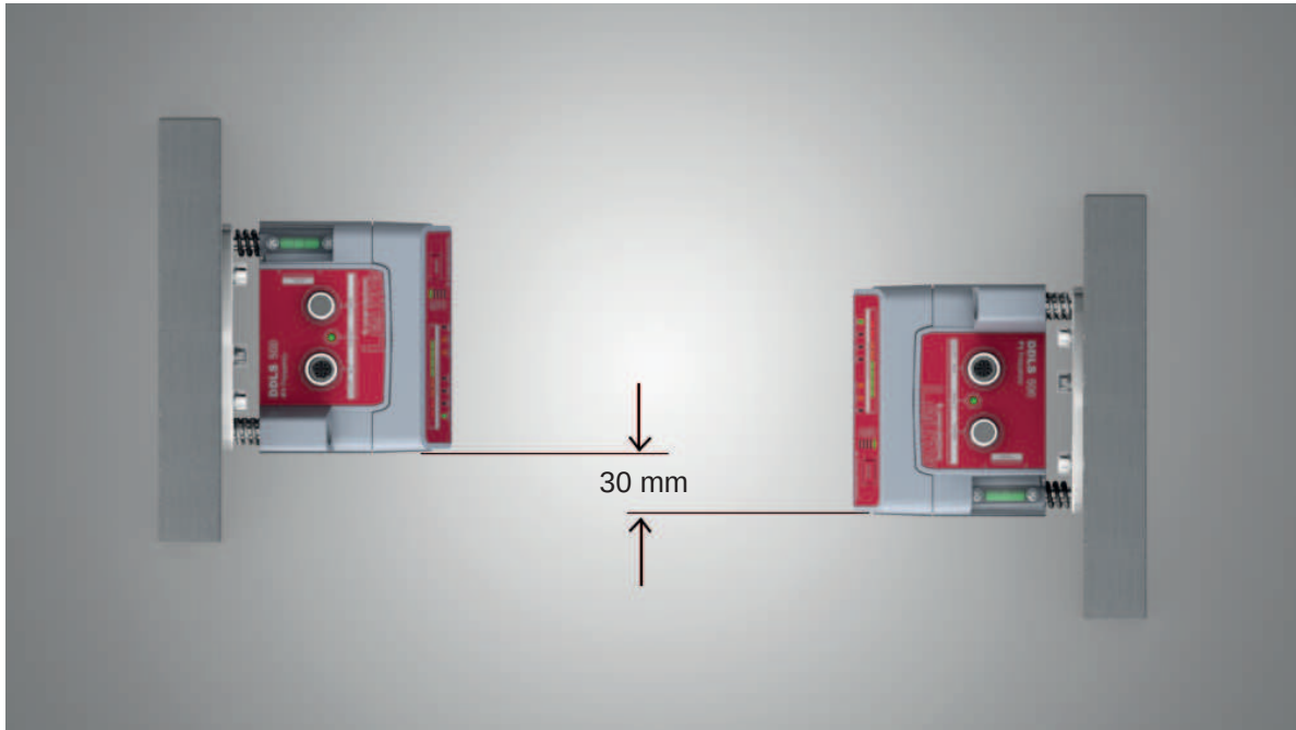
Bild 4.2: Gehäuseversetzte Montage
