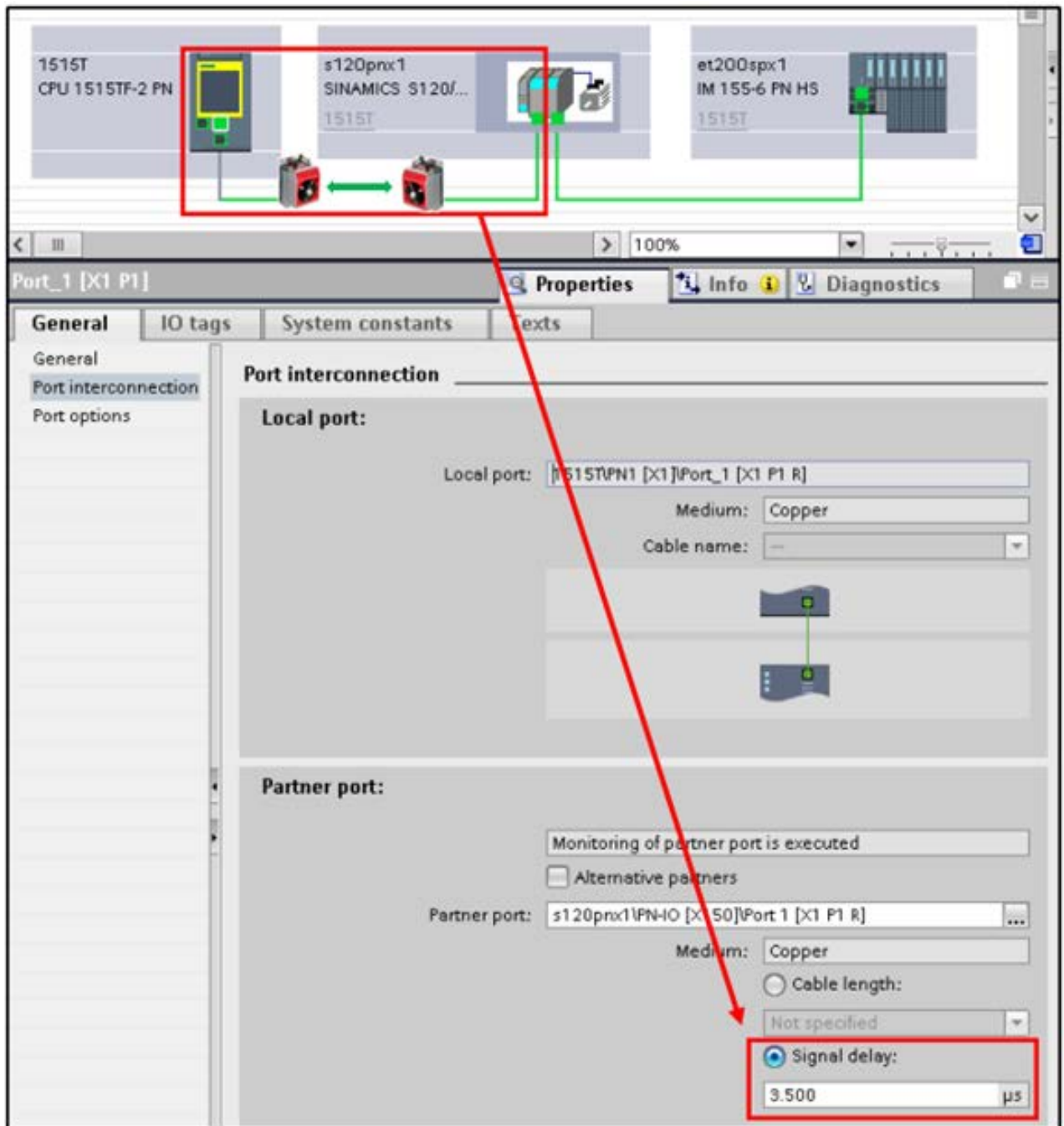
Bild 3.5: Signal delay 3,50 µs
