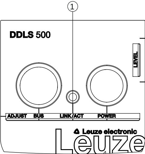
1 LED, Ethernet (geteilt, zweifarbig) LINK/ACT
