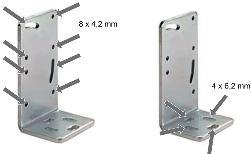
图 10.3: 安装支架 BT 300 W
