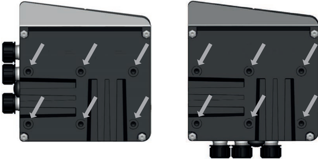
图 10.2: 设备背面的 6 个 M4x5 螺纹孔
