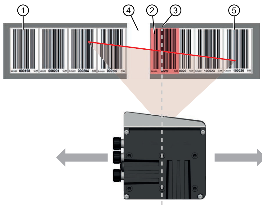
图 9.16: 扫描光束中的数值范围 1 和 2 · 数值范围 1 内贴有 MVS 标签
