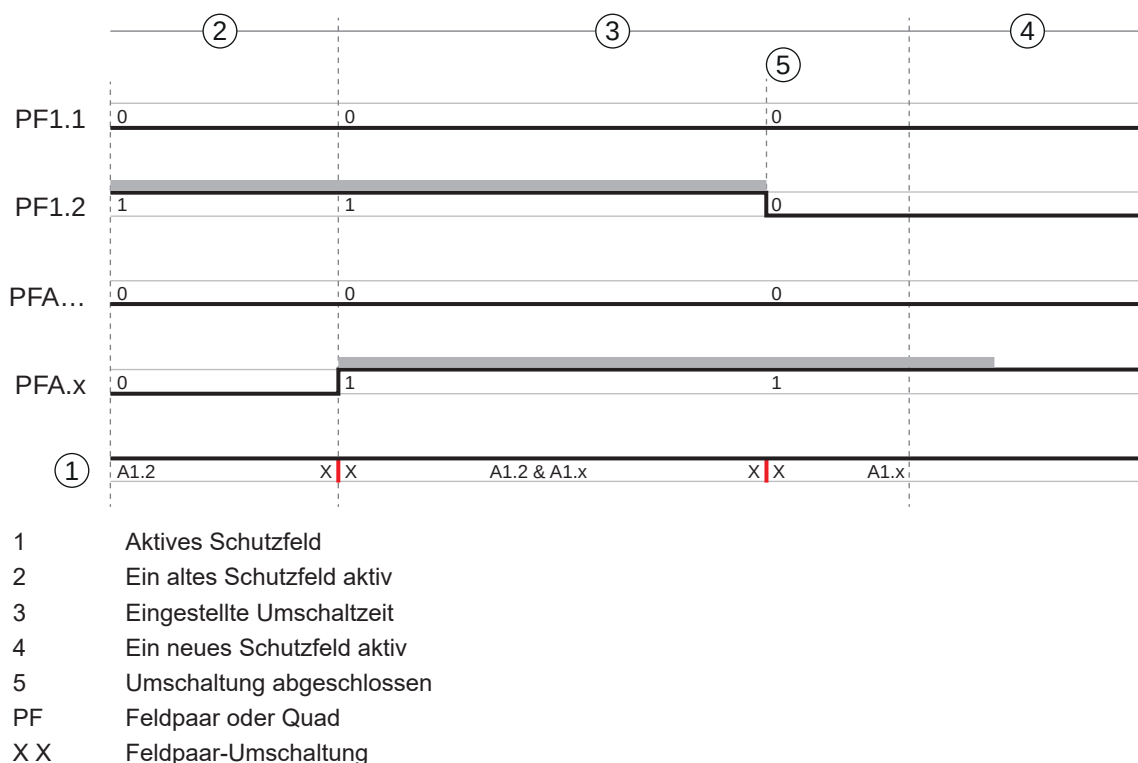
Bild 5.2: Signal-Zeit-Diagramm: Überlappende Überwachung
