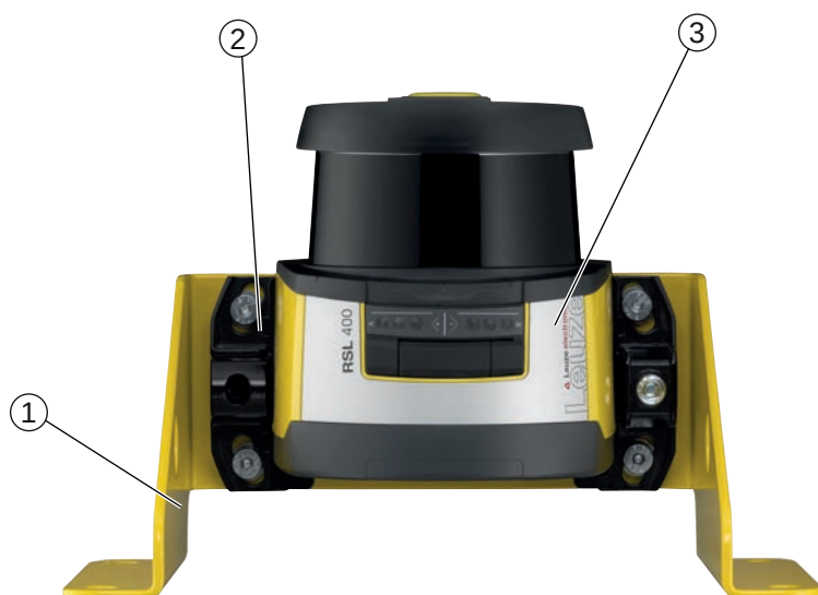
Bild 7.4: Beispiel: Montage an abgeflachter Ecke
