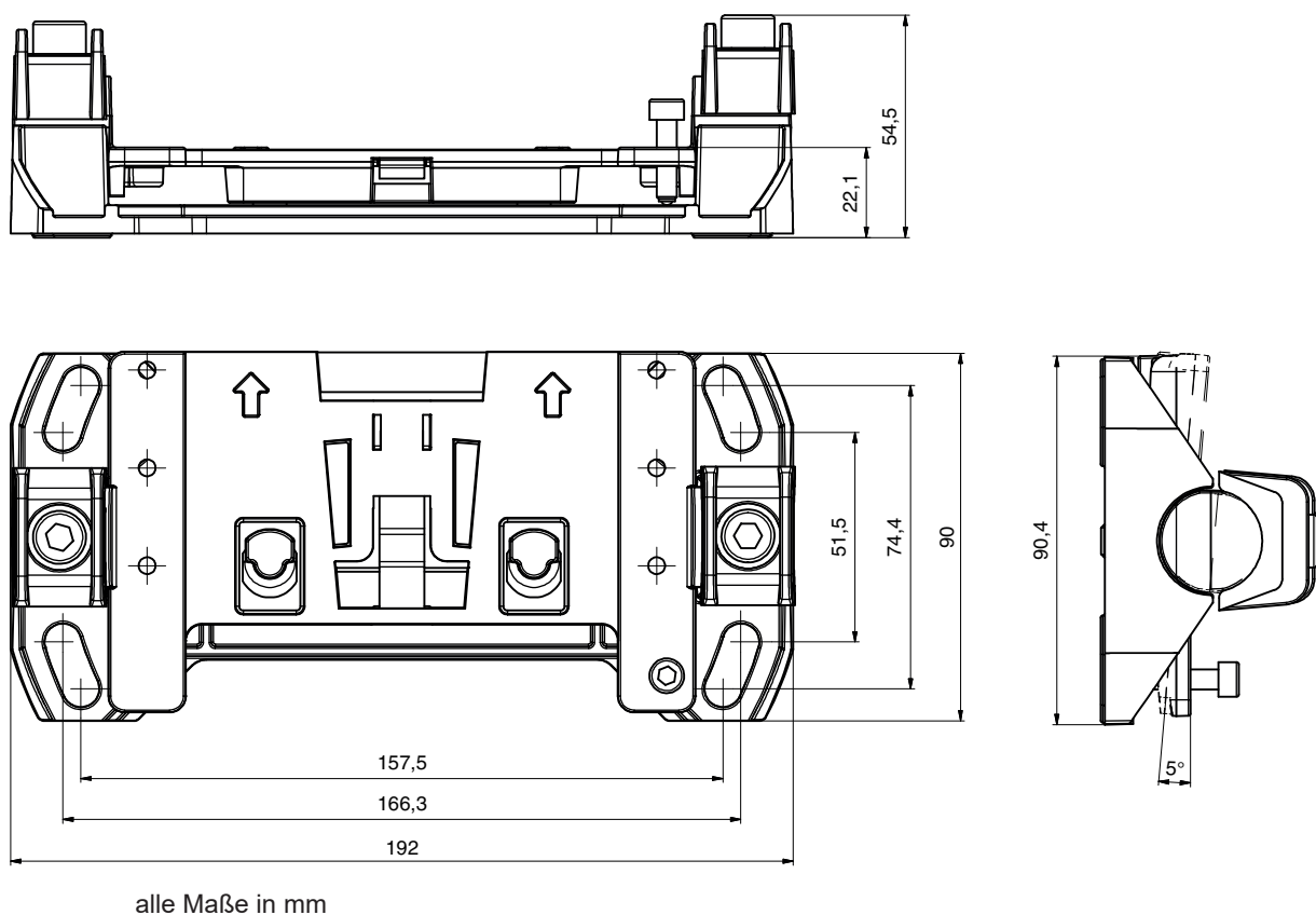
Bild 15.5: Montagesystem BTU800M
