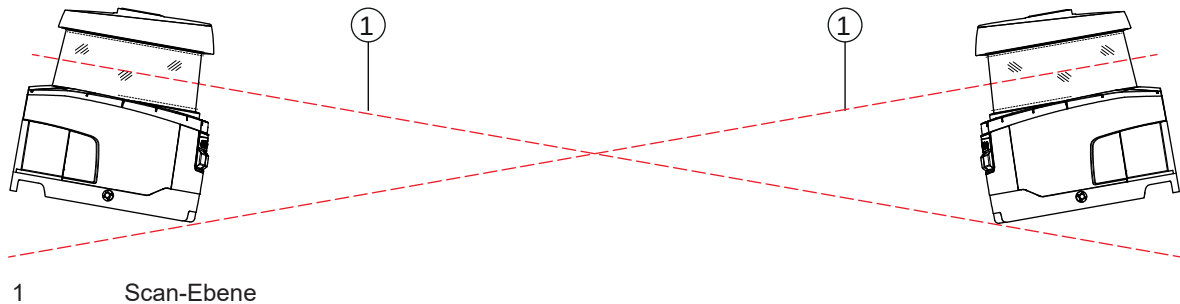
Bild 7.11: Montage gegenüberliegend, ohne Höhenversatz, gekreuzte Ausrichtung
