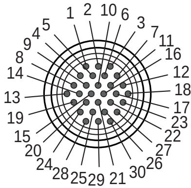
Bild 8.1: Anschlussbelegung M30-Stecker, 30-polig
