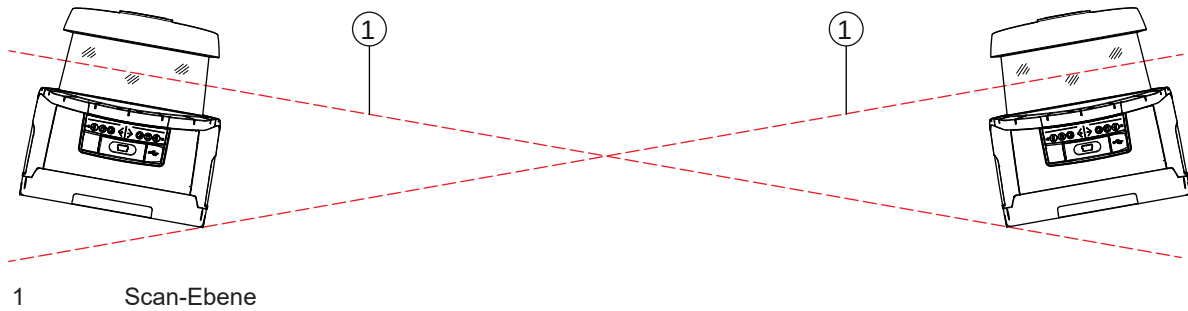
Bild 7.10: Montage nebeneinander, ohne Höhenversatz, gekreuzte Ausrichtung
