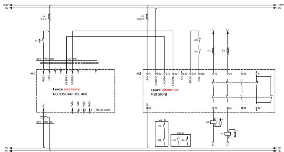
Bild 8.6: RSL 430 mit Sicherheitsrelais MSI-SR4B
