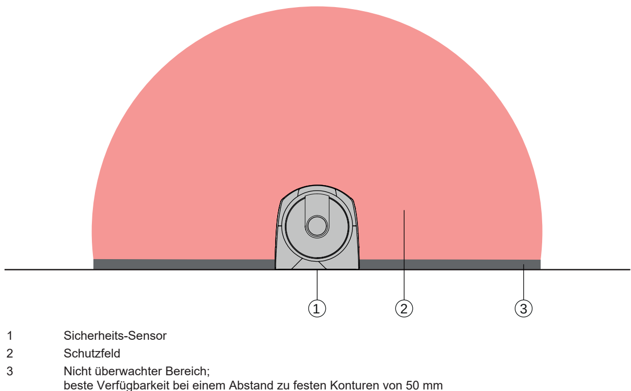
Bild 7.6: Nicht überwachter Bereich
