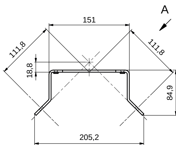
Bild 15.8: Schutzbügel BTP800M
