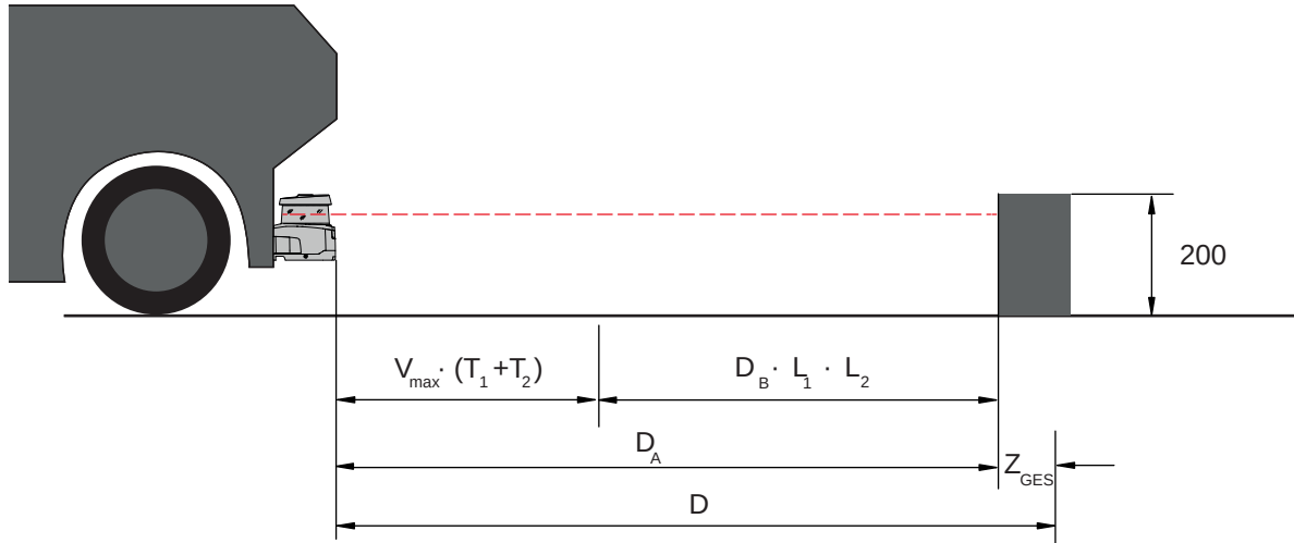
Bild 7.14: Mobile Gefahrenbereichssicherung, Berechnung der erforderlichen Mindestdistanz D
