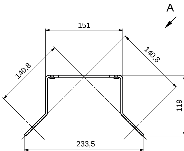
Bild 15.10: Montagewinkel BT840M, Ansicht A
