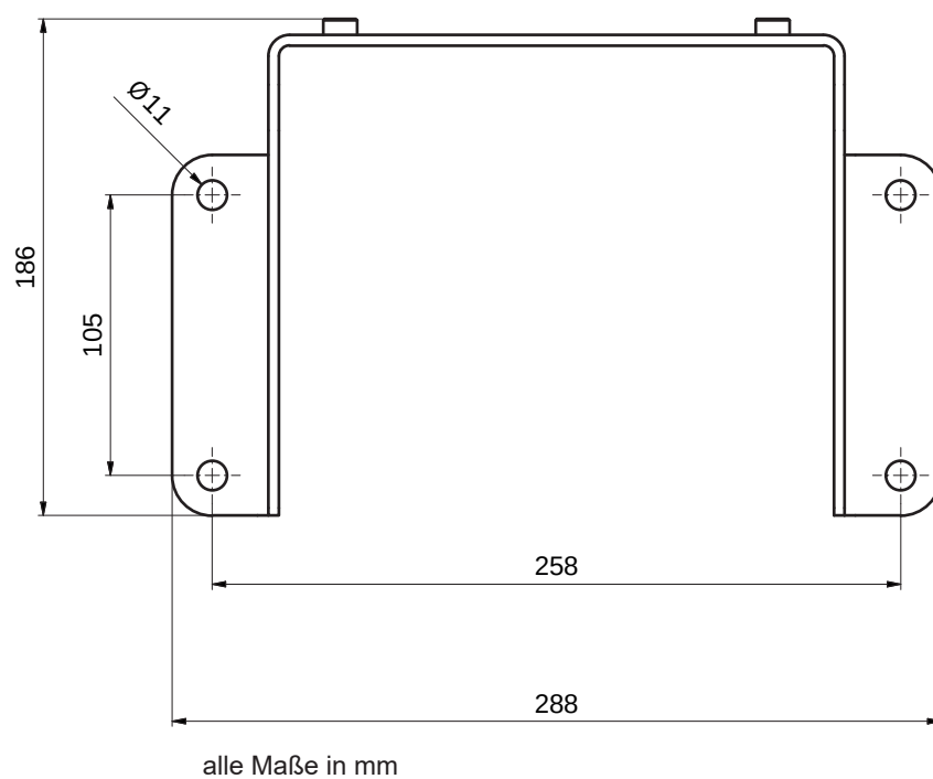
Bild 15.7: Montagewinkel BTF830M
