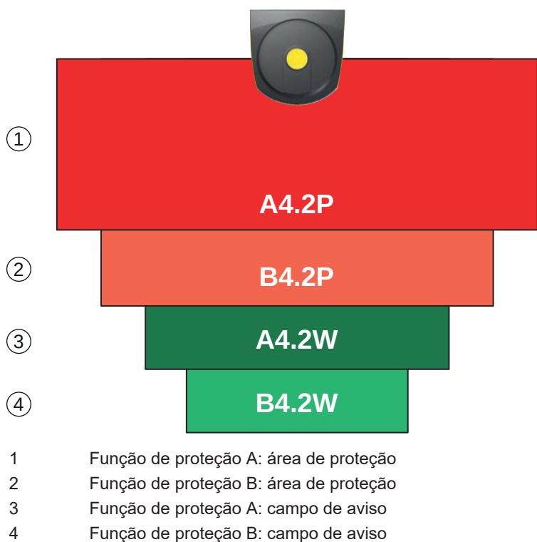
Fig. 5.2: Modo de quatro campos
