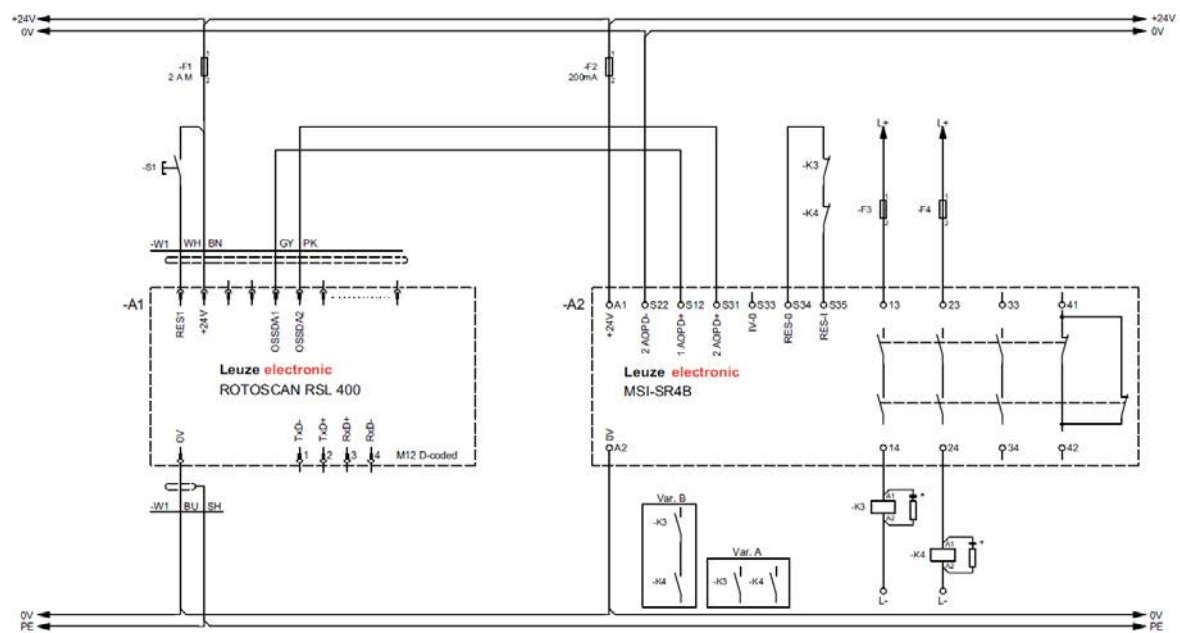
Fig. 8.6: RSL 440 com relé de segurança MSI-SR4B
