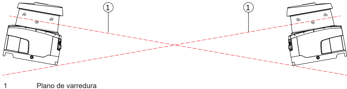
Fig. 7.11: Montagem oposta, sem desfasamento vertical, alinhamento cruzado
