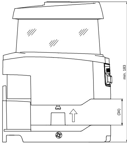
Resim 15.2: Bağlantı ünitesi güvenlik lazer alan tarayıcısı montaj ölçüleri
