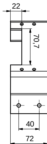
Fig. 15.10: Équerre de montage BT840M, vue A
