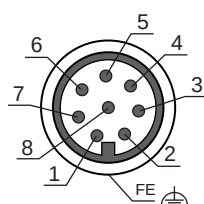
Fig. 8.1: Affectation des raccordements du capteur de sécurité
