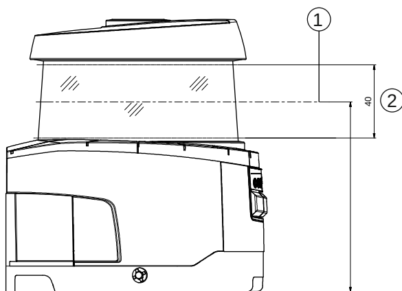
Fig. 7.1: Montage avec prise en compte de la zone de balayage de 270°
