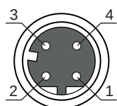
Fig. 8.2: Affectation des raccordements de l'interface Ethernet
