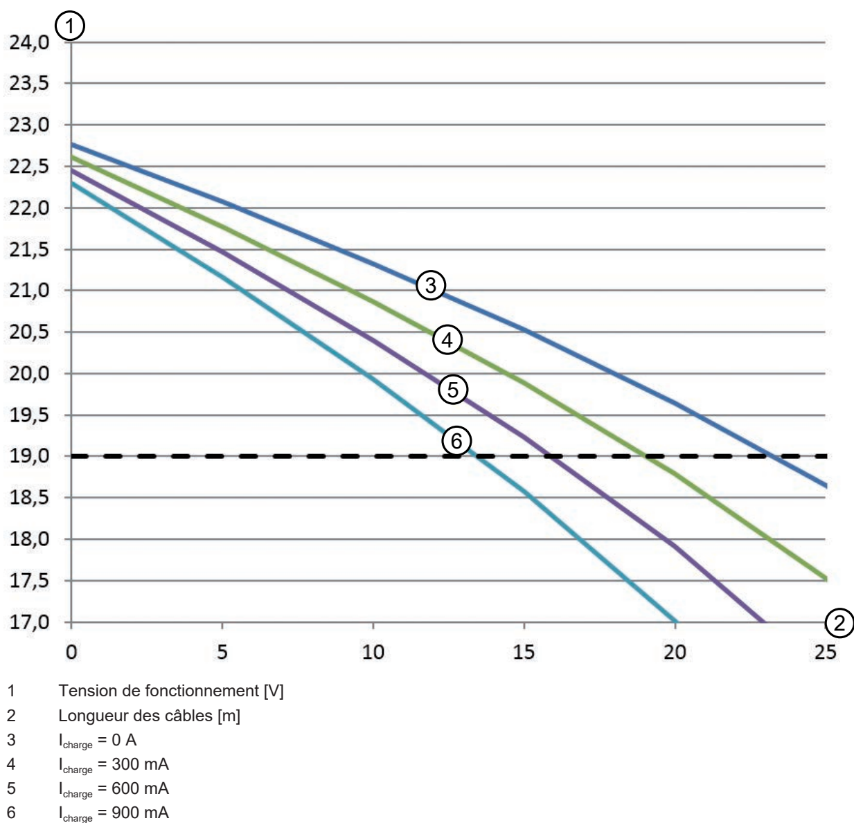
Fig. 8.4: Diagramme d'évaluation de la chute de tension sur la ligne d'alimentation
