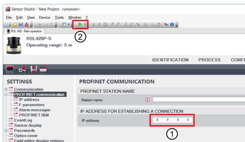
图 4.4: 设备管理器 (DTM) - IP 地址
