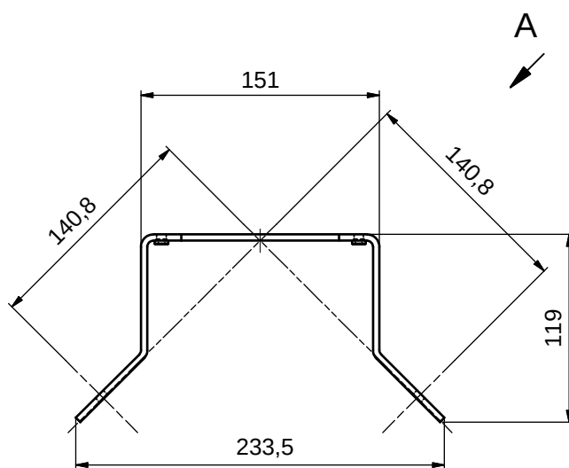
图 16.11: 安装角件 BT840M · 视图 A
