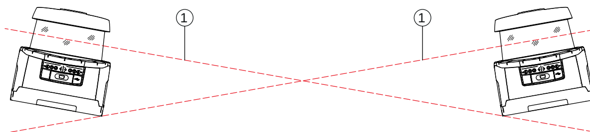
图 7.11: 并排安装 (无高度偏差，带角度偏差)
