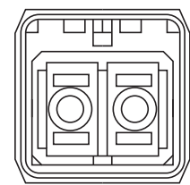
图 8.12: PROFINET SCRJ Push/Pull AIDA 连接
