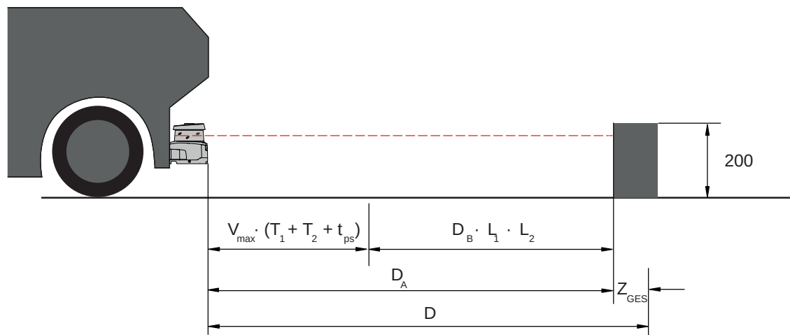
图 7.15: 移动危险区域防护 (计算所需的最小间距 D)
