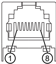
图 8.9: 引线布局 PROFINET RJ45 AIDA-Push/Pull
