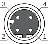
图 8.3: 引线布局 M12 插口 · 4 针 · D 编码
