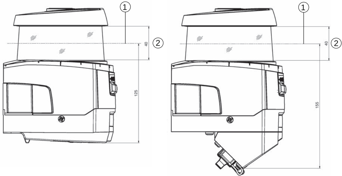
图 7.1: 考虑 270° 的扫描范围进行安装
