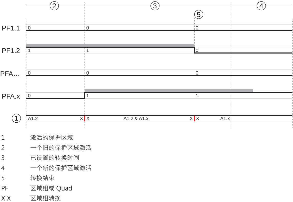
图 5.2: 信号时间图：重叠监控
