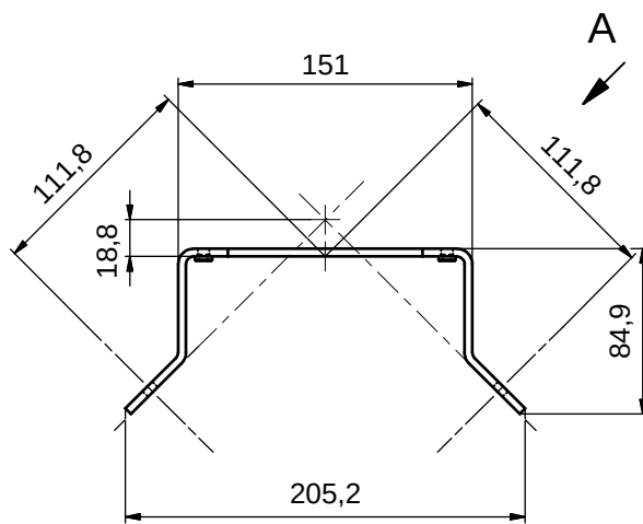
图 16.9: 防护栏 BTP800M
