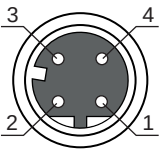
图 8.6: 引线布局 M12 插口 · 4 针 · D 编码
