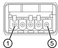
图 8.11: 引线布局 PROFINET AIDA Push/Pull · 5 针
