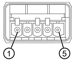
图 8.8: 引线布局 PROFINET AIDA Push/Pull · 5 针
