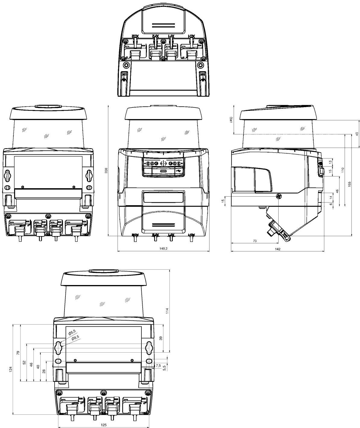
图 16.3: 安全激光扫描仪的尺寸，含连接单元 CU400P-4M12、CU400P-AIDA 或 CU400P-AIDA-OF
