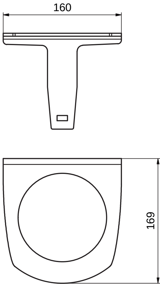
图 16.9: 防护栏 BTP800M
