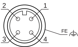
图 8.2: 引线布局 M12 插口 · 4 针 · A 编码
