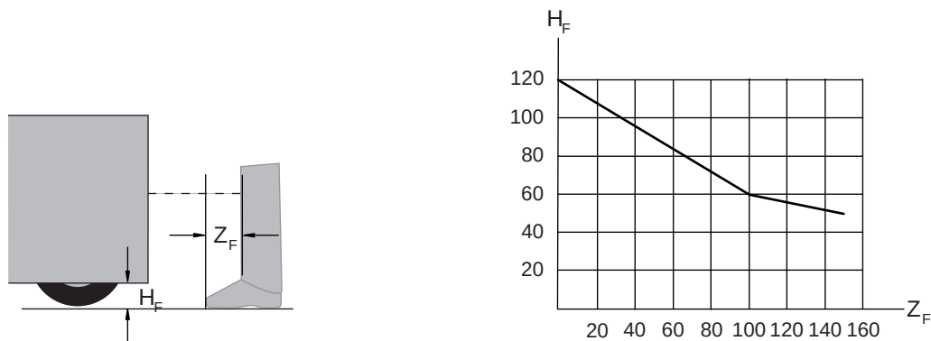
图 7.16: 用于确定附加值 Z_F 的图标（离地高度 H_F 不够）
