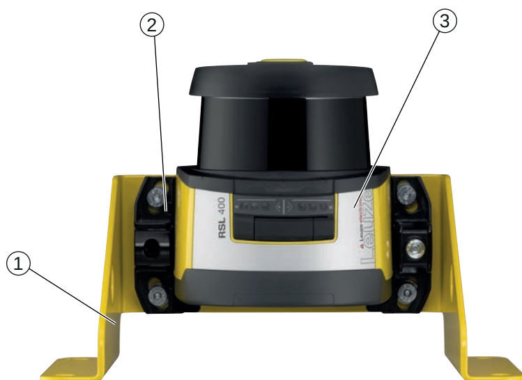
图 7.5: 示例：在扁平角上安装
