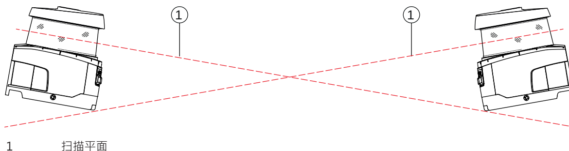
图 7.12: 相对安装 (无高度偏差, 带角度偏差)
