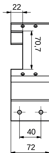
图 16.11: 安装角件 BT840M · 视图 A
