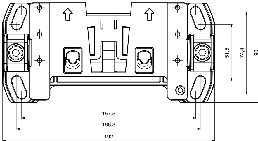
图 16.5: 安装系统 BTU800M
