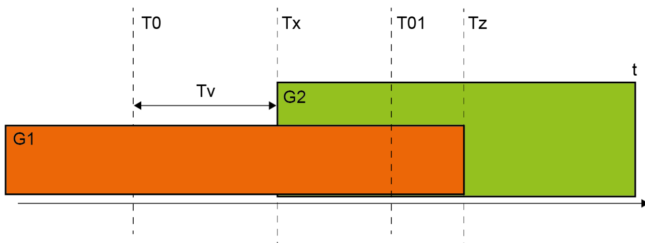
图 5.15: 2 个危险位置的保护区切换
