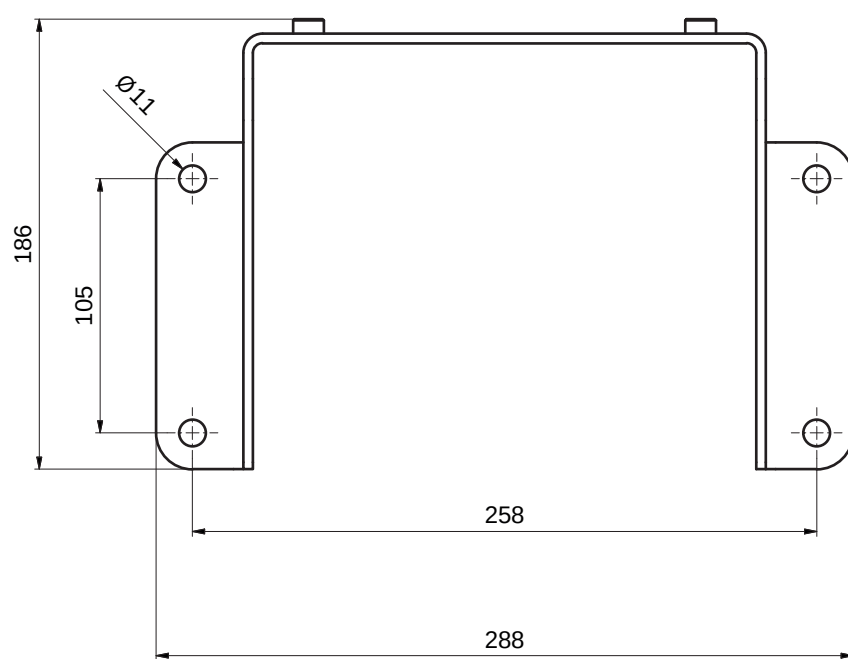
图 16.8: 安装角钢 BTF830M
