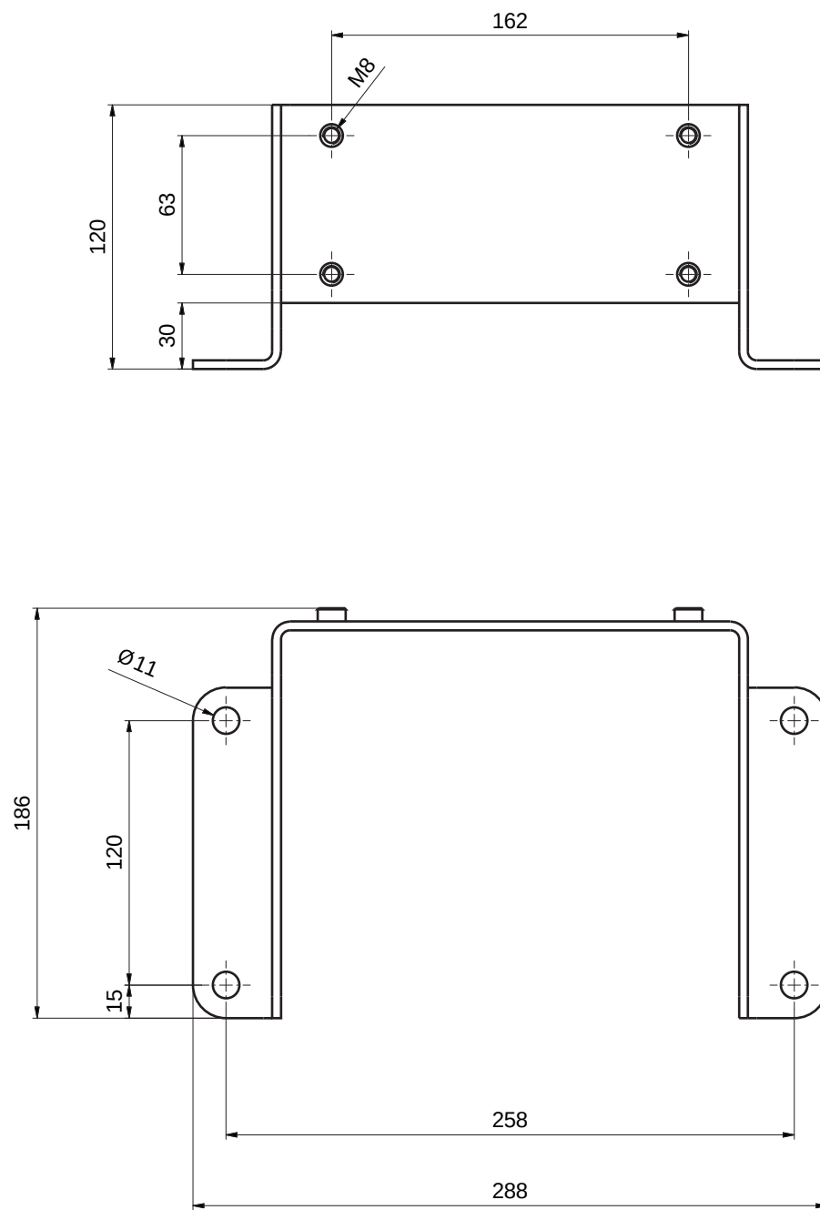
图 16.7: 安装角钢 BTF815M
