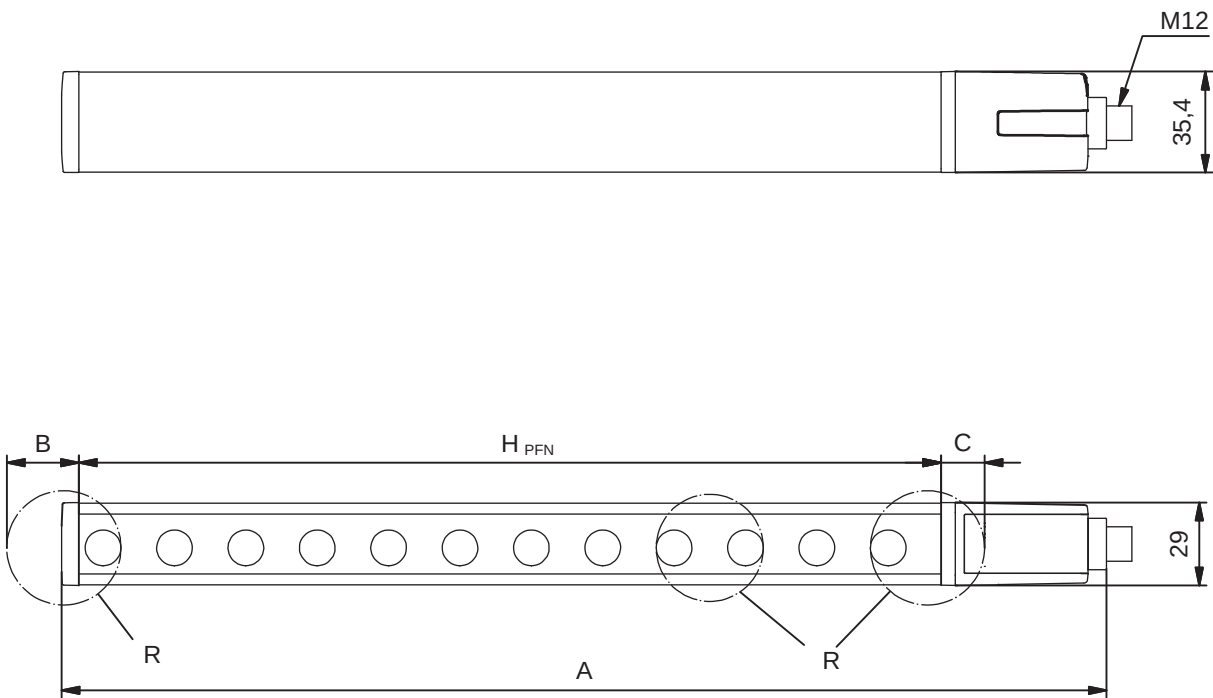
Fig. 14.1: Dimensions de l'émetteur et du récepteur La hauteur effective du champ de protection H_{PFE} va au-delà des dimensions de la zone optique jusqu'aux arêtes extérieures des cercles signalés par la lettre « R ».
