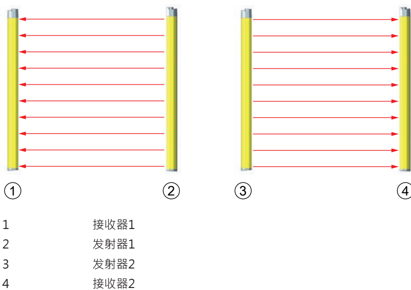
图 6.5: 背向安装
