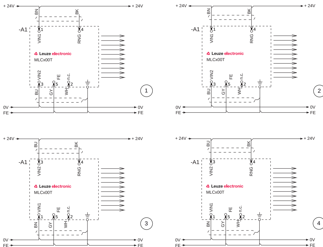
Bild 7.2: Anschlussbeispiele Sender
