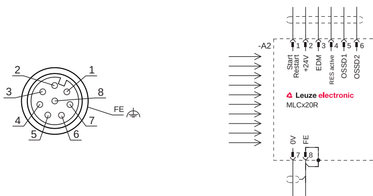
Bild 7.3: Steckerbelegung und Anschlussbild Empfänger
