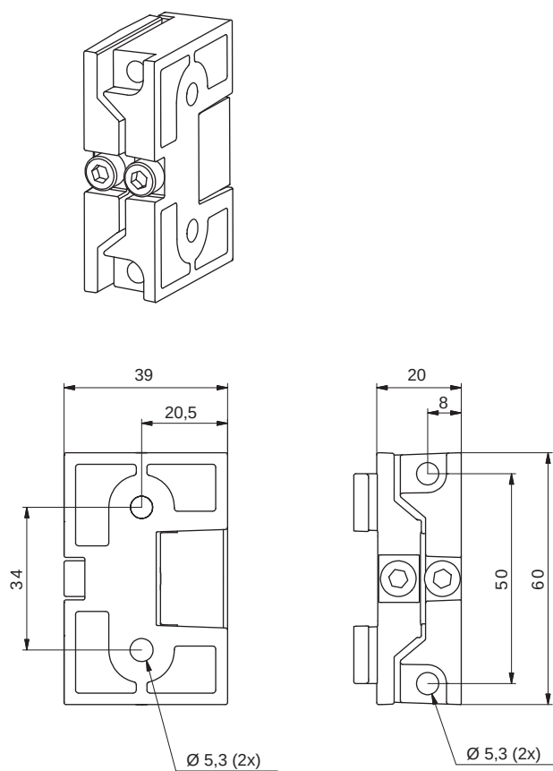
Bild 14.5: Schwenkhalterung BT-2SB10
