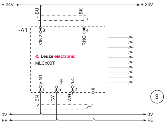
图 7.2: 发射器连接示例
