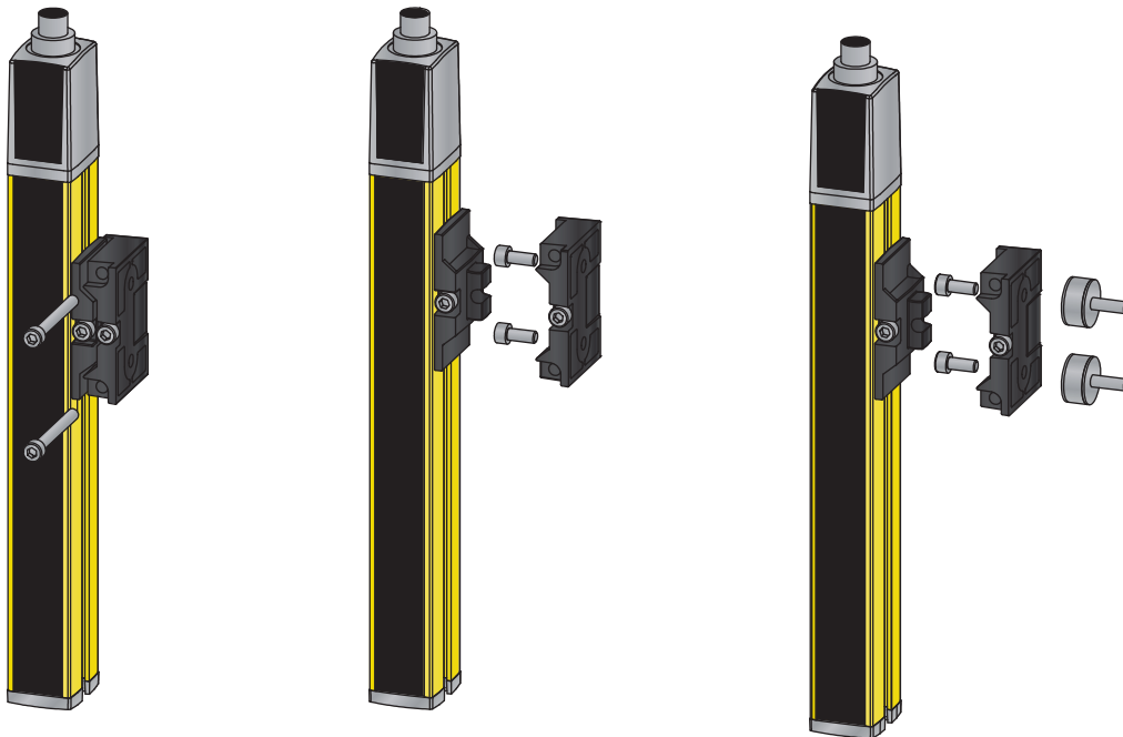
Figura 6.9: Montaggio mediante supporti orientabili BT-2SB10
