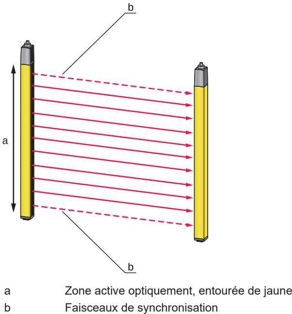
Fig. 3.1: Système émetteur-récepteur
