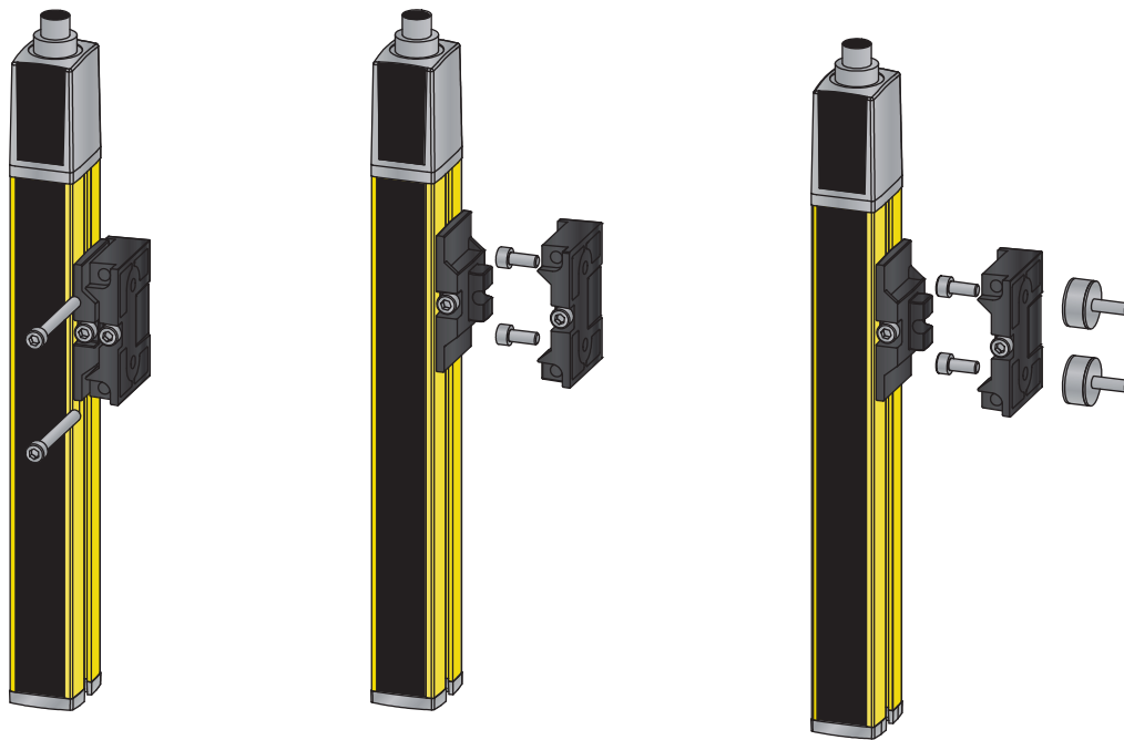
Figura 6.9: Montaggio mediante supporti orientabili BT-2SB10
