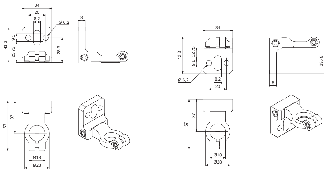
图 15.5: 转座 BT-2HF
