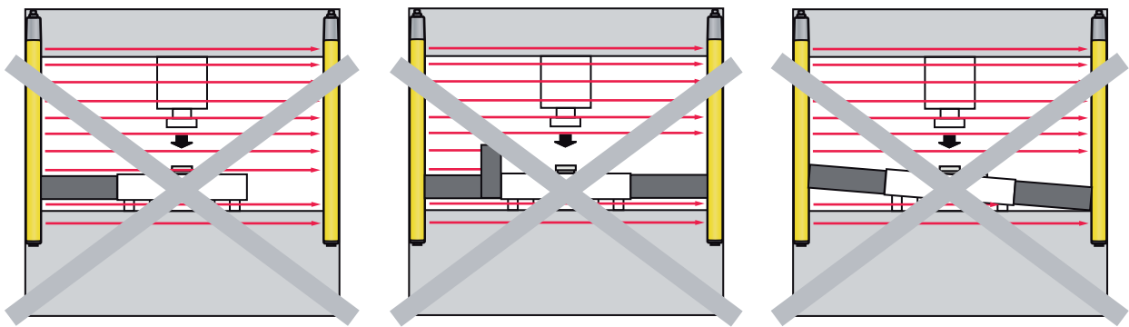
图 5.3: 固定消隐：避免产生阴影
