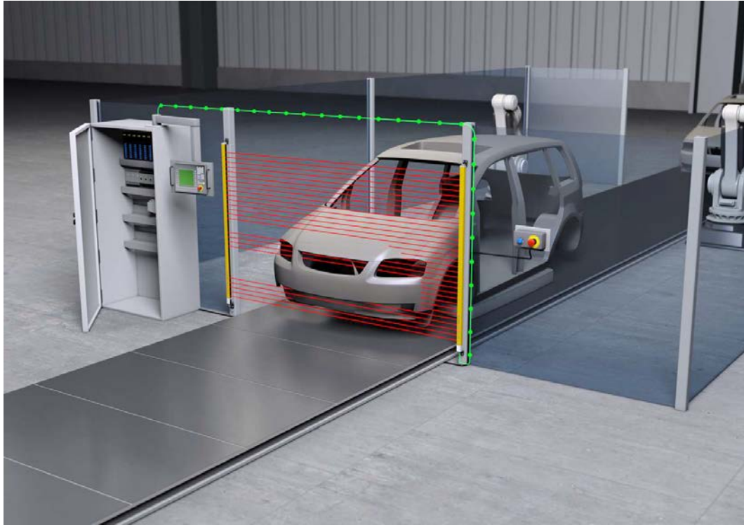
图 6.1: Kfz 生产线上的智能过程门控 (SPG)
