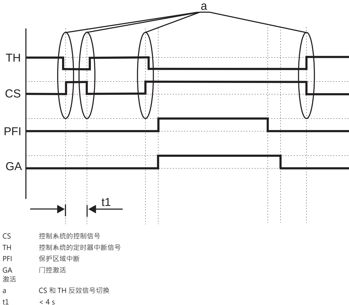
图 4.3: 运行模式1 - 合格的停止
