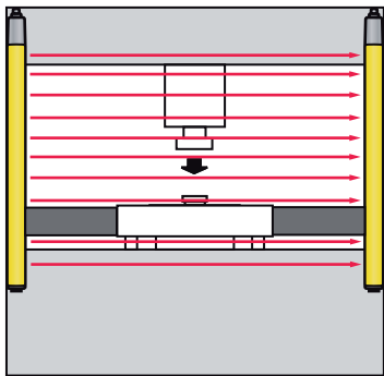
图 5.2: 固定消隐：机械锁止件防止从侧面进入保护区域 保护区域内不能形成阴影。
