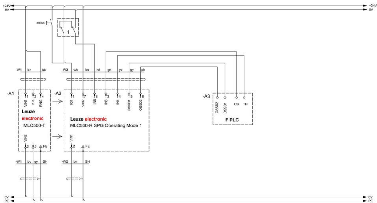
图 8.4: 运行模式 1：含智能过程门控 (SPG) 的连接示范
