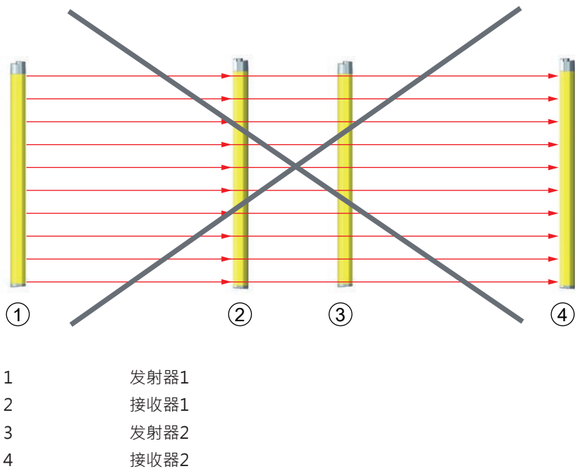
图 7.4: 不当安装导致相邻安全传感器之间产生光学串扰（发射器1影响接收器2）
