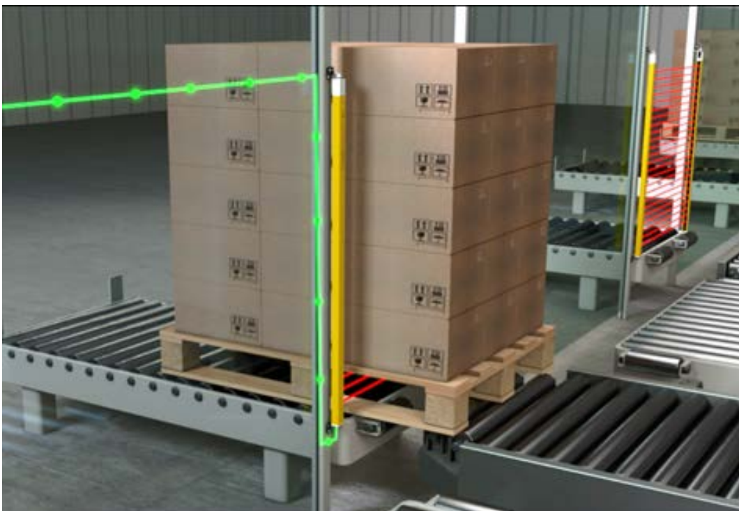
图 6.2: 输送线上的智能过程门控 (SPG)
