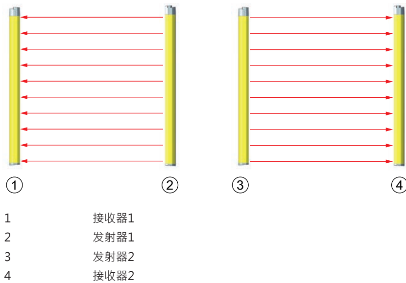
图 7.5: 背向安装
