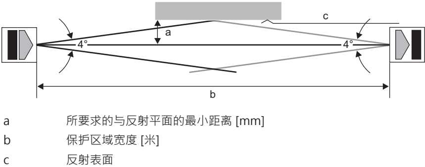
图 6.2: 根据保护区域的宽度决定的与反射平面的最小距离
