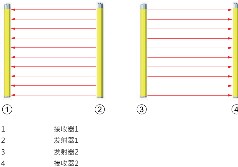
图 6.5: 背向安装
