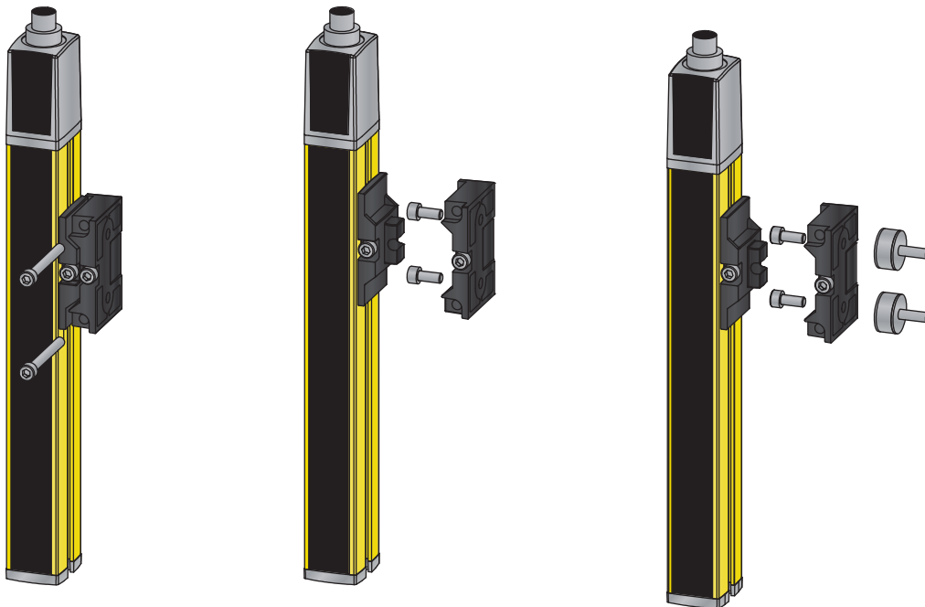
图 6.9: 通过可转动支架 BT-2SB10 安装
