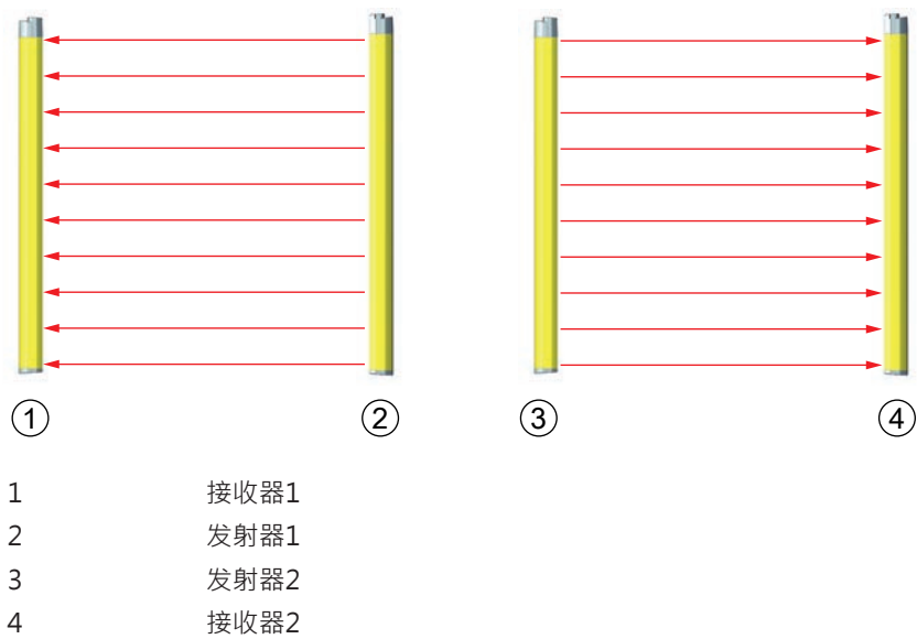
图 6.5: 背向安装
