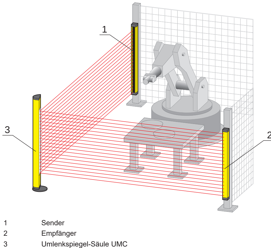
Bild 6.12: Anordnung mit Umlenkspiegel-Säule zur 2-seitigen Absicherung einer Gefahrstelle
