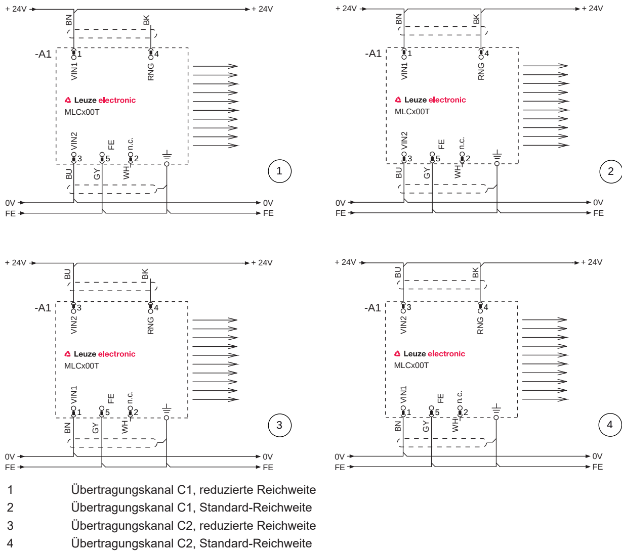
Bild 7.2: Anschlussbeispiele Sender
