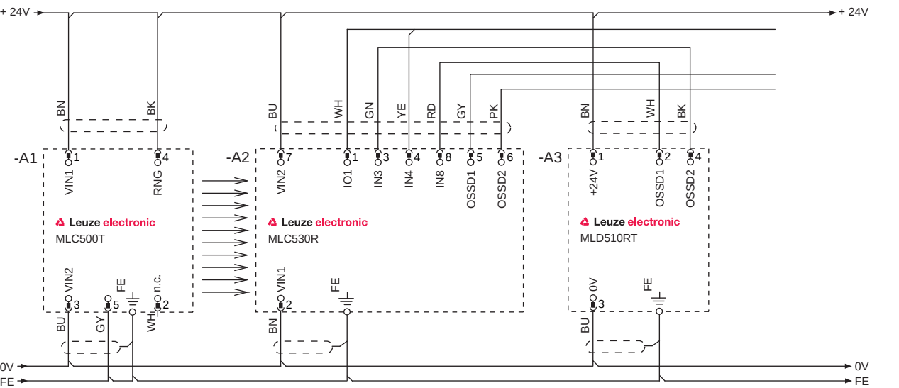
图 7.7: 运行模式2：联接了电子安全开关输出端的接线示例，用于门禁和危险区域组合防护
