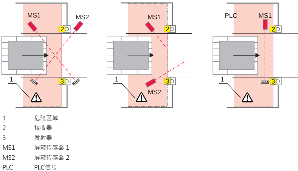
图 6.9: 定时双传感器屏蔽在驶出应用中的屏蔽传感器布置
