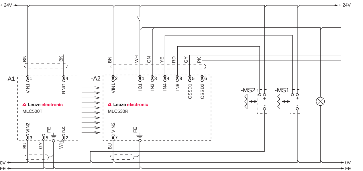
图 7.13: 运行模式6：定时双传感器屏蔽（局部）的接线示例
