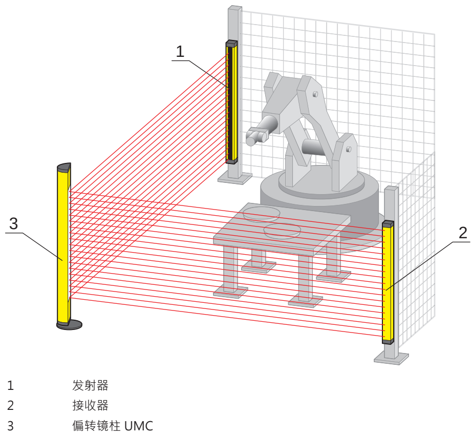
图 6.18: 通过偏转镜柱实现双面防护
