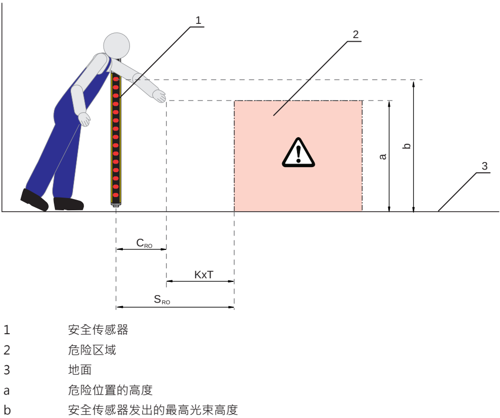
图 6.1: 有爬行或跨越进入可能性时的安全距离的附加值
