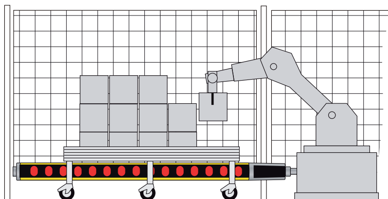
图 4.4: 分辨率降低；多个小物体可同时在保护区域内移动或从保护区域中取出
