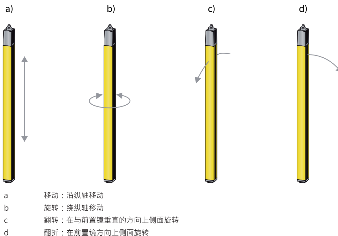
图 6.10: 校准安全传感器的移动方向
