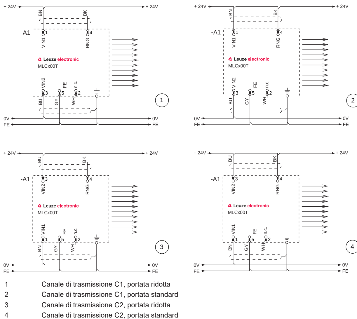
Figura 7.2: Esempi di collegamento del trasmettitore
