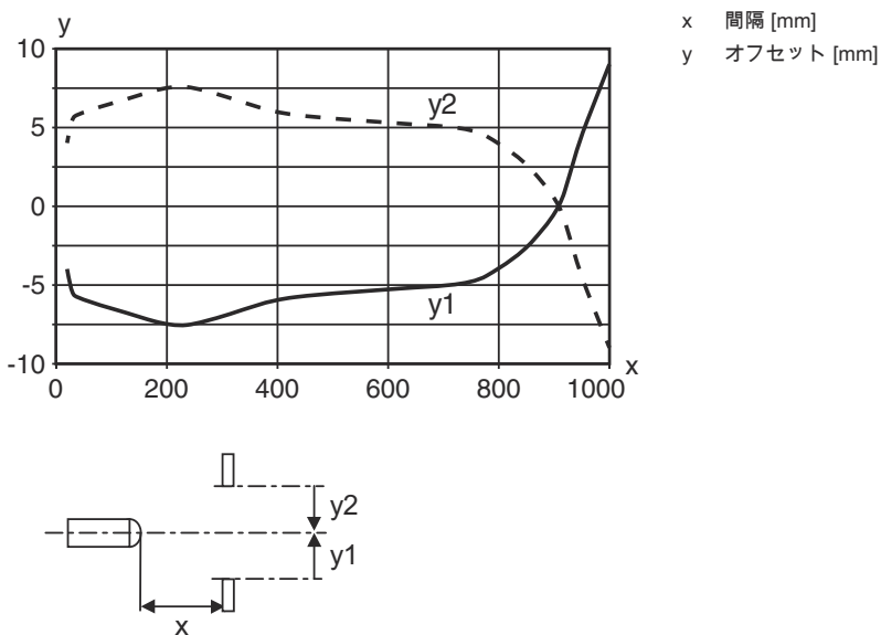
典型的応答挙動 (調整距離 1000mm)
