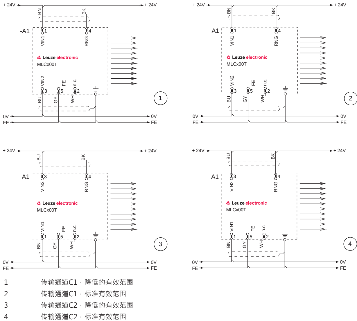
图 7.3: 发射器连接示例
