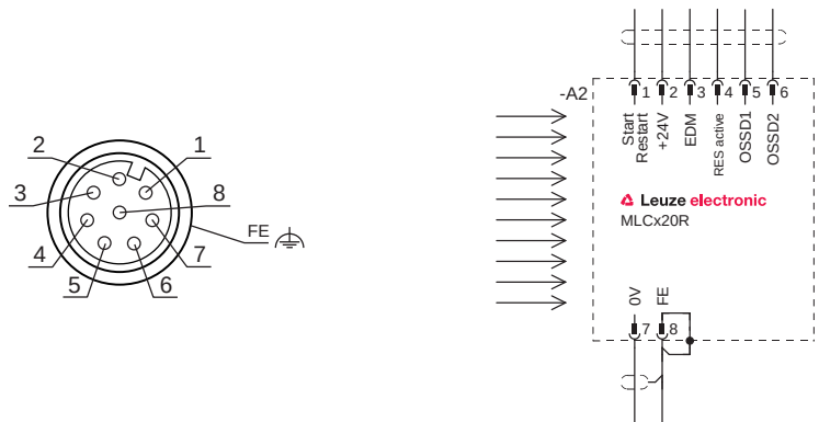
图 7.4: 接收器的插头分配和接线图
