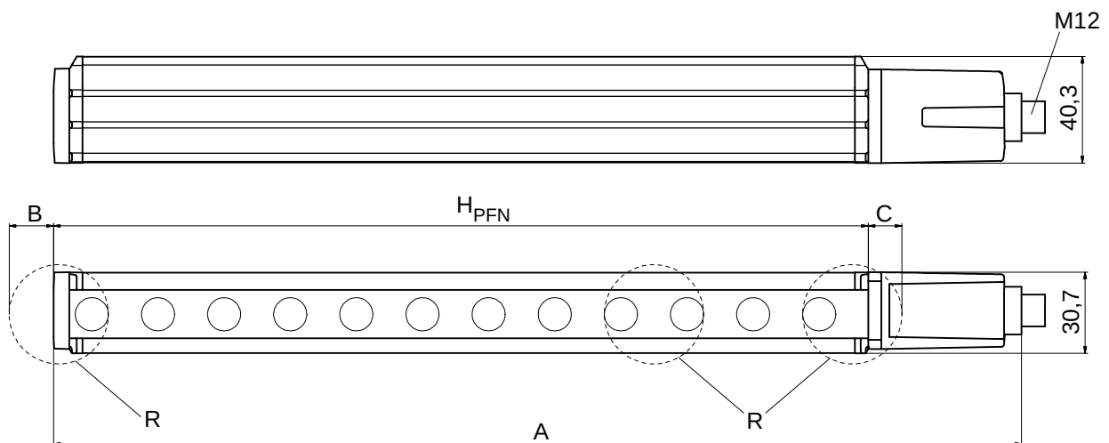
Fig. 14.1: Dimensions de l'émetteur et du récepteur
