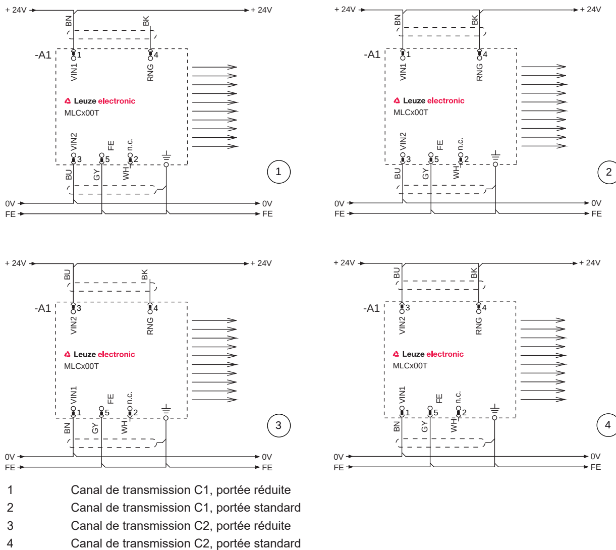
Fig. 7.3: Exemples de branchement de l'émetteur
