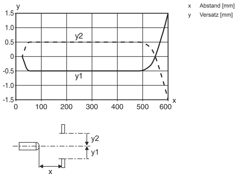
Typ. Ansprechverhalten (Einstellentfernung 600 mm)
