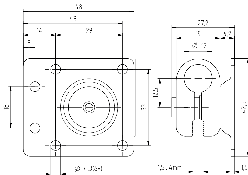
Figura 15.3: Dibujo acotado del sistema de montaje BTU 320M-D12
