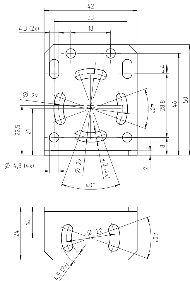
Figura 15.4: Dibujo acotado de escuadra de fijación BT 320M
