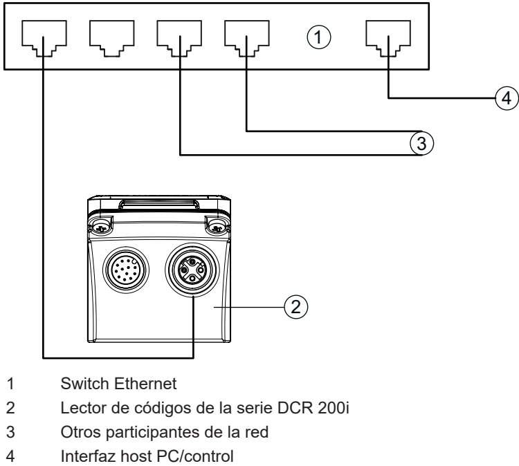
Figura 7.6: Topologías de estrella Ethernet
