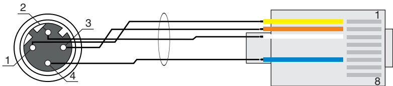
Figura 7.7: Asignación de cables HOST en RJ-45
