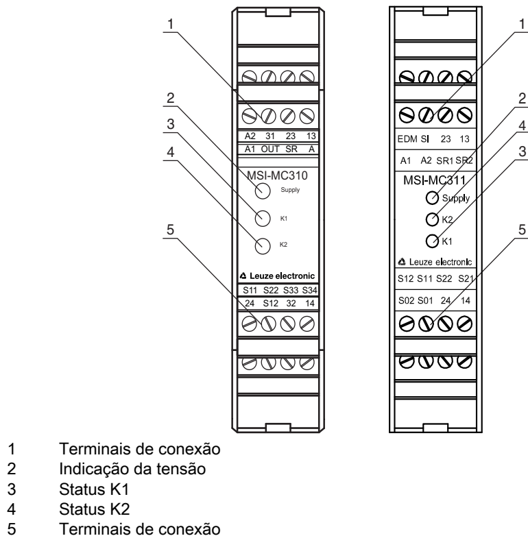
Ilustração 3.5: Relé de segurança MSI-MC310 e MSI-MC311
