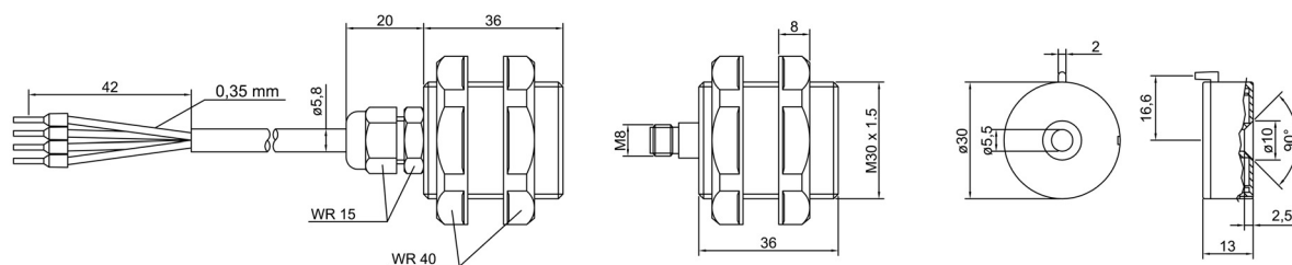
Ilustração 15.3: Dimensões do sensor MC330x e atuador
