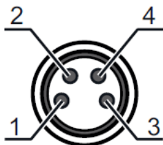
Ilustração 7.7: Pinagem do conector M8 (4 polos)
