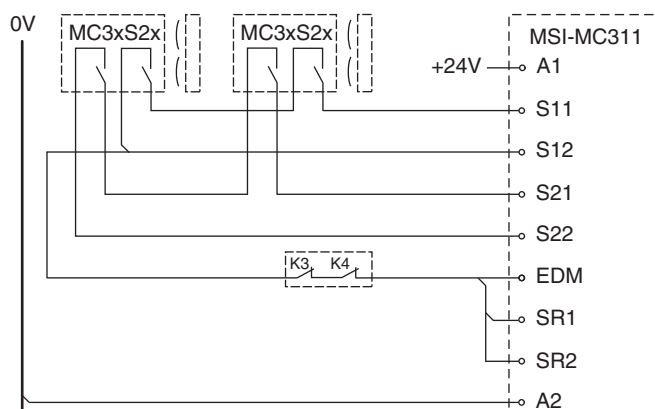
Ilustração 7.15: Exemplo 2: conexão de dois MC3xS2x com inicialização/rearme automático e monitoramento do contator (EDM), representação dos contatos sem ativação pelo atuador
