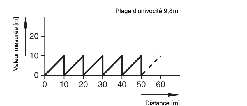
Figure 3.10 : Valeurs de mesure de l'ODSL 30 pour une plage d'univocité de 9,8m
