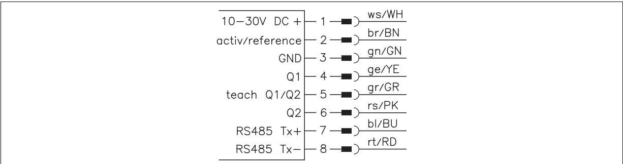
Figure 4.5 : Raccordement électrique de l'ODSL 30/D 485...
