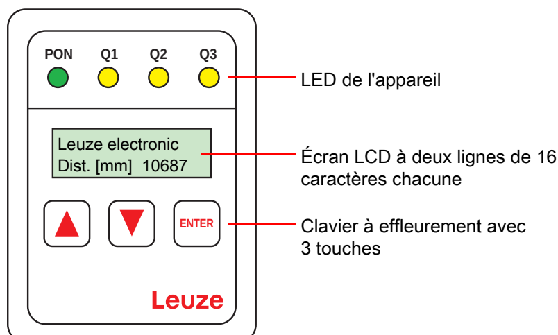
Figure 3.9 : Éléments d'affichage et de commande de l'ODSL 30
