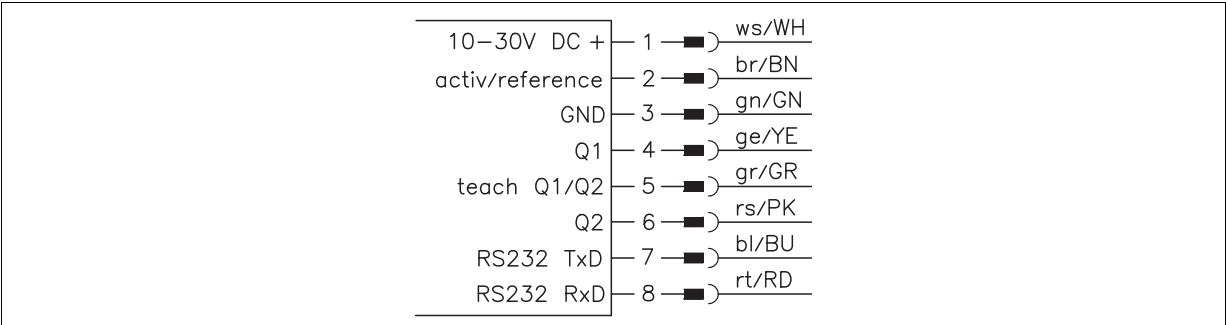
Figure 4.4 : Raccordement électrique de l'ODSL 30/D 232...
