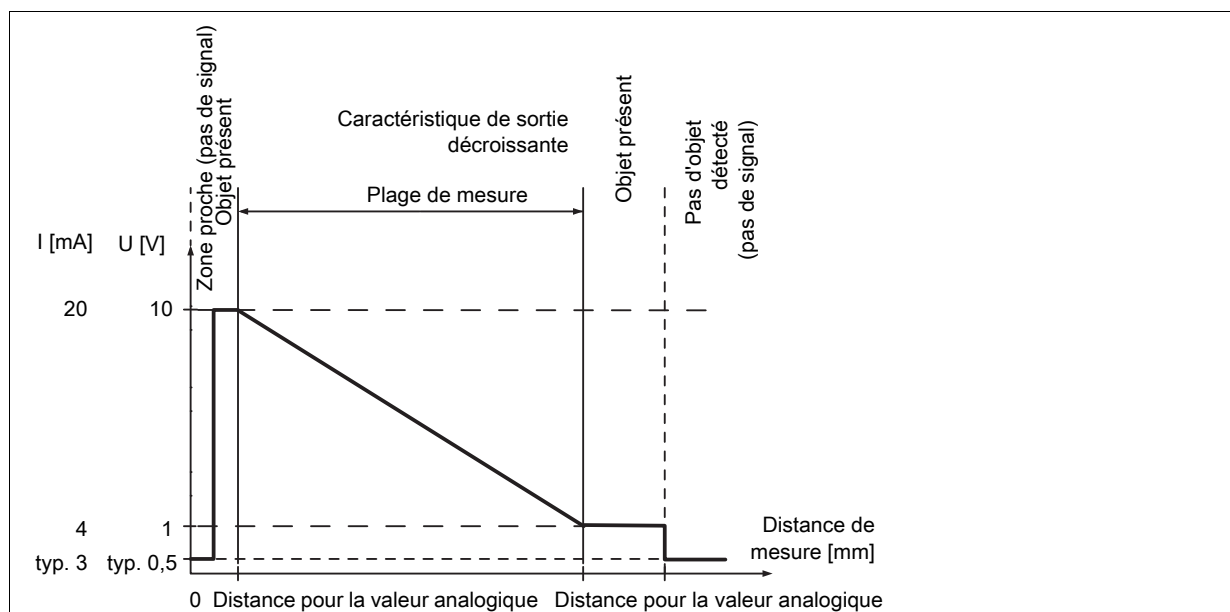
Figure 3.5 : Caractéristique de sortie ODSL 30/V... de pente négative
