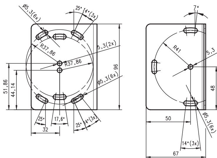
Figure 3.3 : Encombrement de la pièce BT 30
