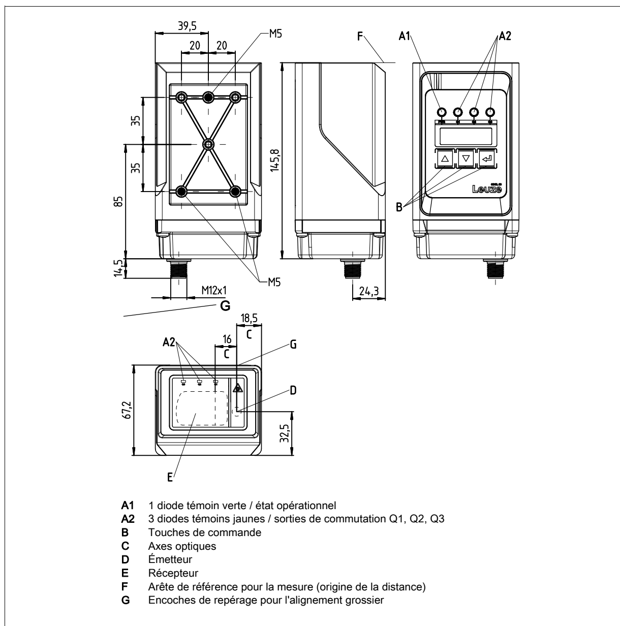
Figure 4.1 : Encombrement des différents ODSL 30
