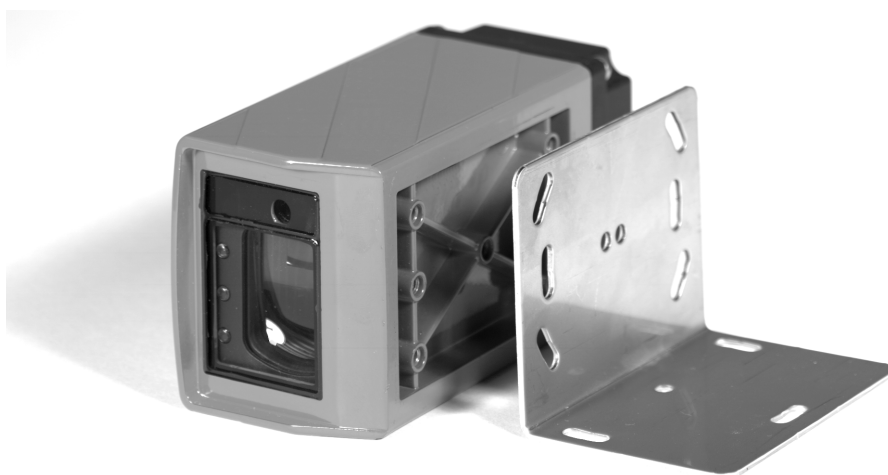
Figure 3.2 : ODSL 30 et BT 30
