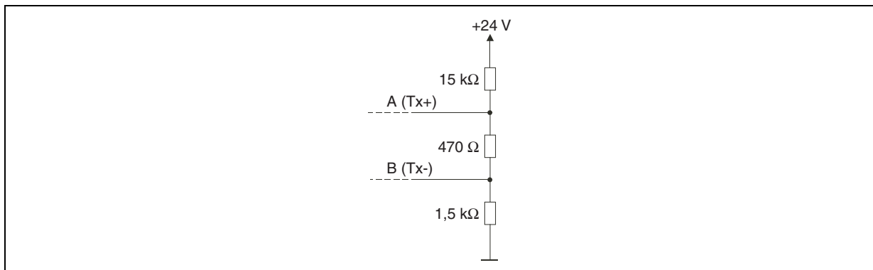
Figure 3.8 : Diviseur de tension pour la terminaison du bus RS 485
