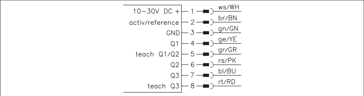
Figure 4.3 : Raccordement électrique de l'ODSL 30/24...
