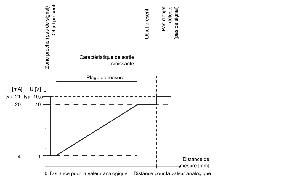
Figure 3.4 : Caractéristique de sortie ODSL 30/V... de pente positive
