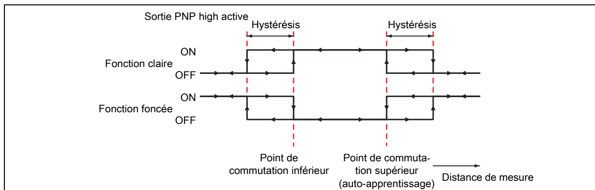
Figure 3.6 : Comportement des sorties de commutation ODSL 30/24... (sortie PNP high active)
