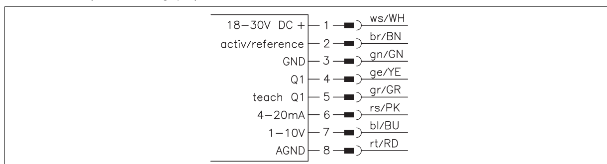
Figure 4.2 : Raccordement électrique de l'ODSL 30/V...
